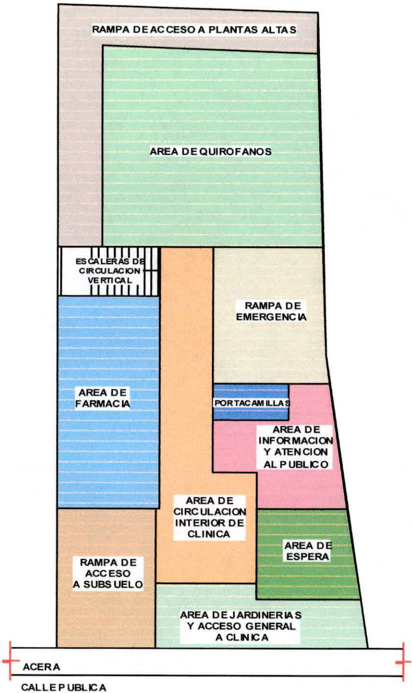
PLANTA DISTRIBUCION FUNCIONAL EN PLANTA BAJA DE CLINICA Y UBICACION DE FARMACIA
