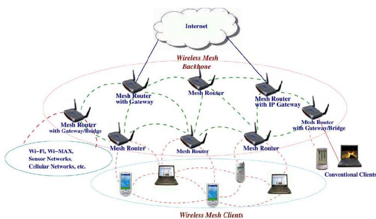
Figura 2-9 Red WMN Híbrida.
