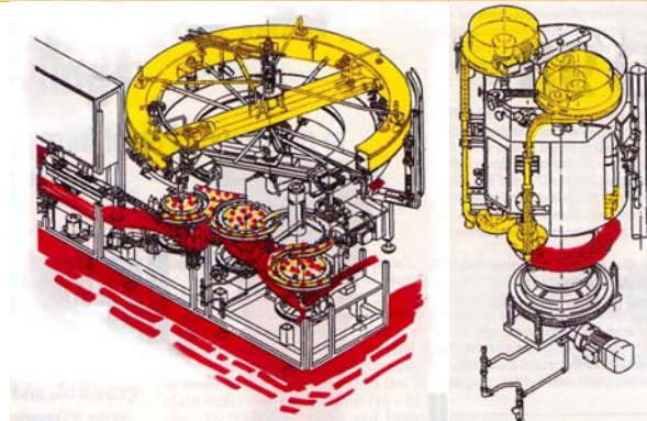
Zonas de riesgo en una envasadora
