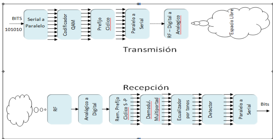
Fig 3. Representación de diagrama de bloques del sistema completo OFDM usando ecualización por tonos
