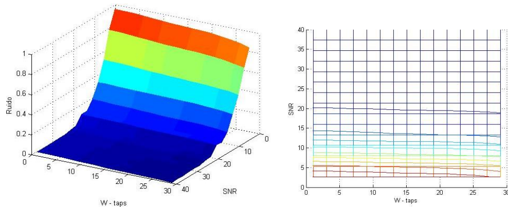
Fig 10. Gráfica SNR, Numero Tap,y el Ruido remanente con filtro de orden 30 máximo junto a sus líneas de nivel
