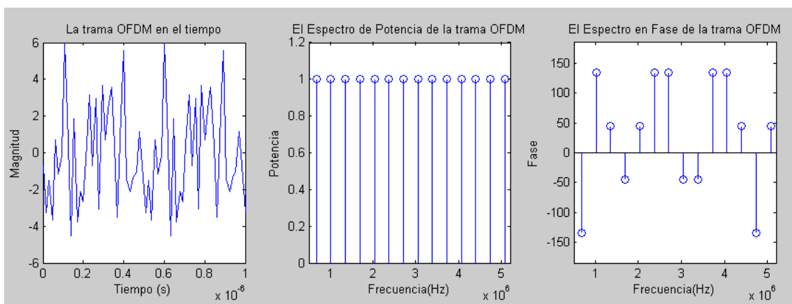
Fig4. Simulación de cada tono (subportadora) en el tiempo junto con la gráfica de símbolos que representa cada un, nótese la desviación en fase presente en cada subportadora
