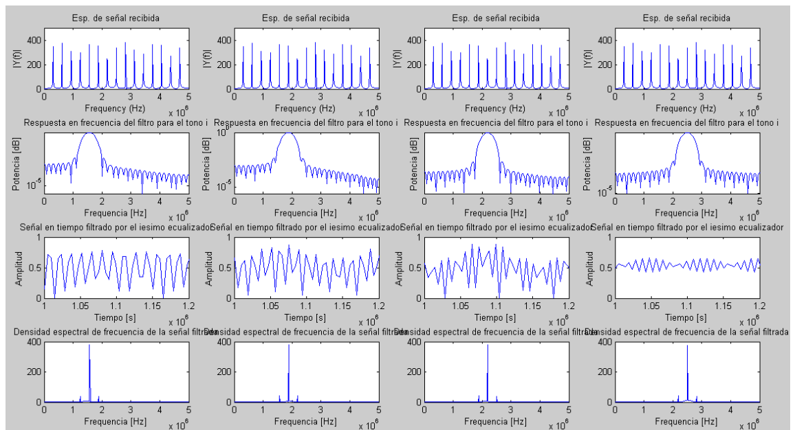
Fig 8. Simulación de los tonos 4, 5,6, y 7 aplicando un w de 60, existen aun pequeñas componentes en las vecindades del i -ésimo tono
