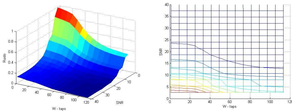
Fig 11. Gráfica SNR, Numero Tap,y el Ruido remanente con filtro de orden 110 máximo junto a sus líneas de nivel
