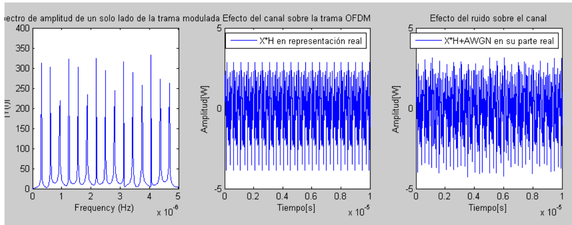
Fig 6. Espectro de frecuencia de la señal aun en el transmisor, efecto del canal sobre la señal en tiempo y efecto del ruido
