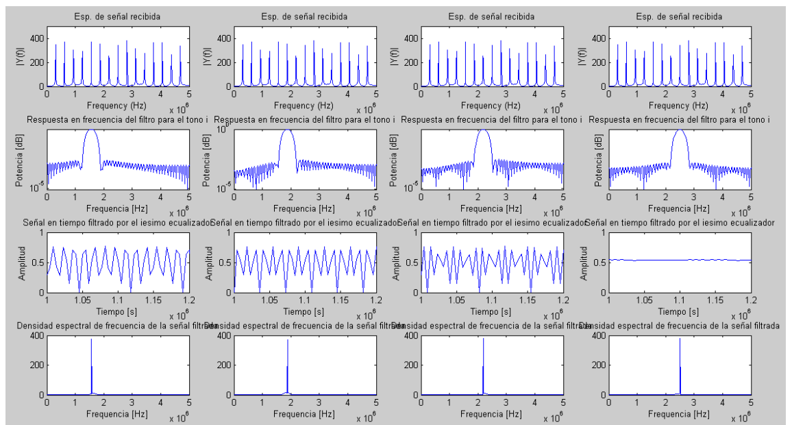
Fig 9. Simulación de los tonos 4, 5,6, y 7 aplicando un w de 100, se puede observar que las componentes espectrales vecinas han desaparecido
