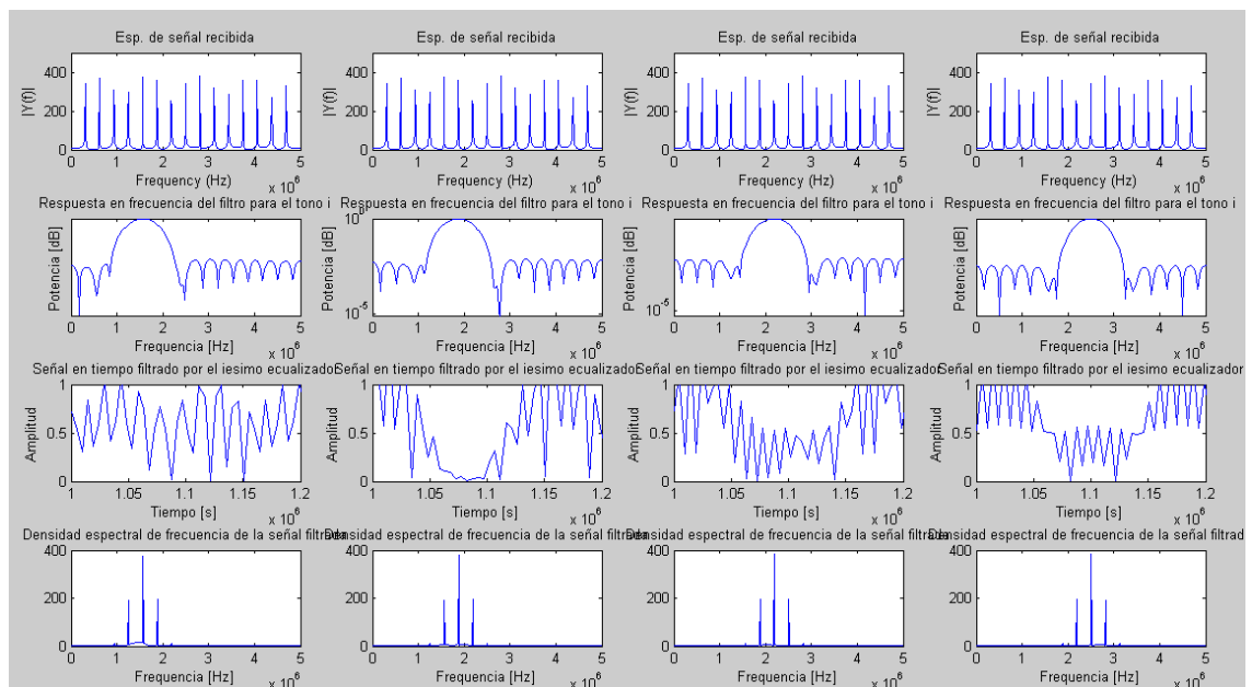
Fig 7 Simulación de los tonos 4, 5,6, y 7 aplicando un w de 30, se puede observar que aun se encuentran en la señal filtrada aun componentes espectrales de las subportadoras vecinas
