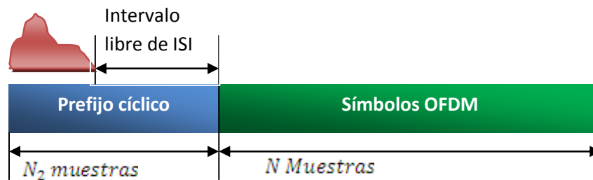
Fig.1 Representación del efecto del prefijo cíclico
