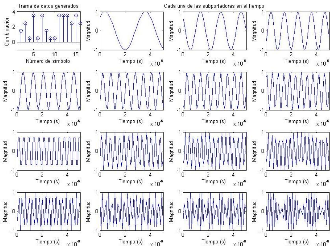
Fig4. Simulación de cada tono (subportadora) en el tiempo junto con la gráfica de símbolos que representa cada un, nótese la desviación en fase presente en cada subportadora
