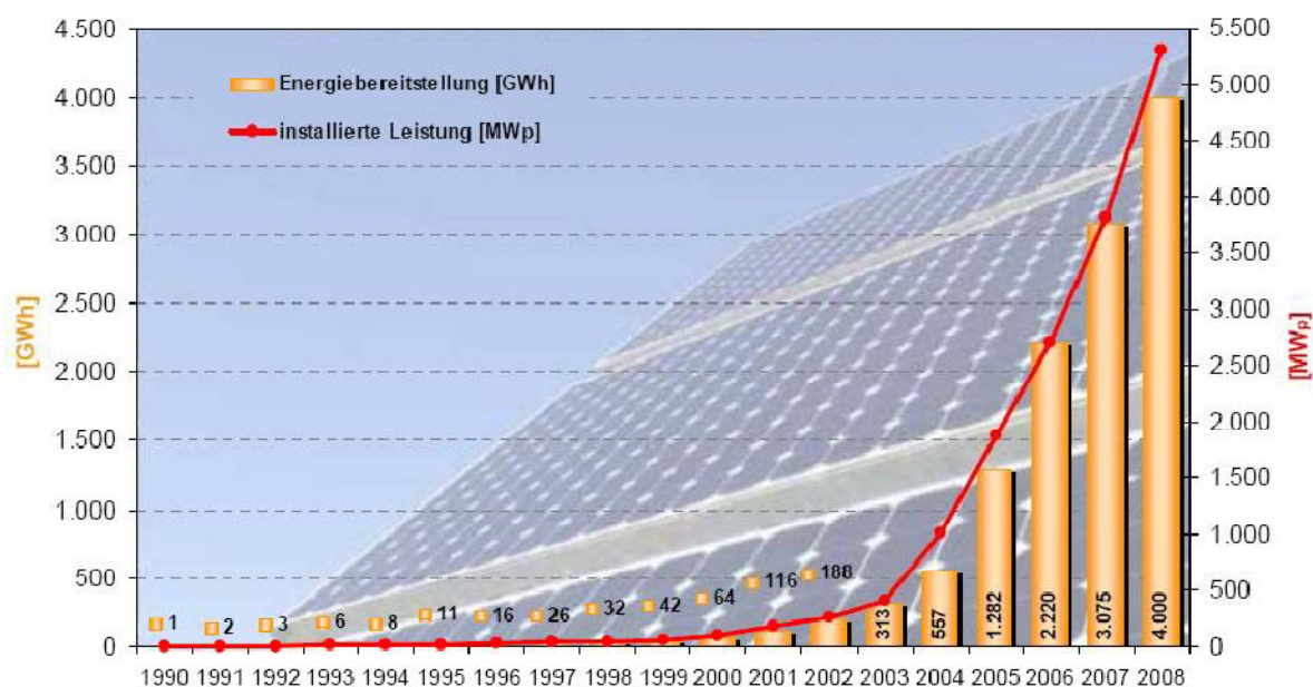
Figura 2.6. Potencia instalada y rendimiento anual de instalaciones fotovoltaicas entre 1990 y 2008
