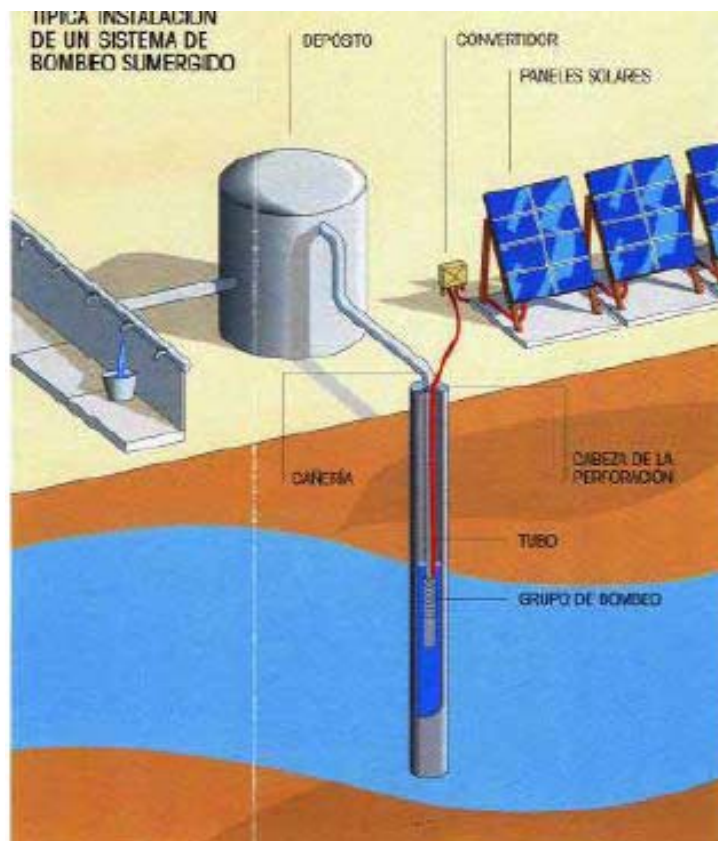
Figura 3.9. Sistema de Bombeo de Agua Fotovoltaico
