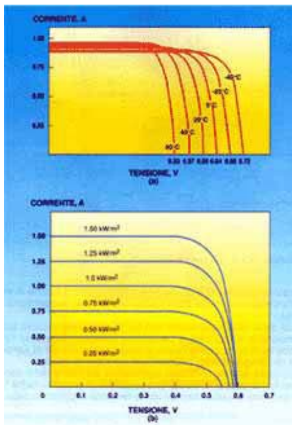
Figura 3.12a. Propiedades Tensión vs. Corriente de Módulos Fotovoltaicos
