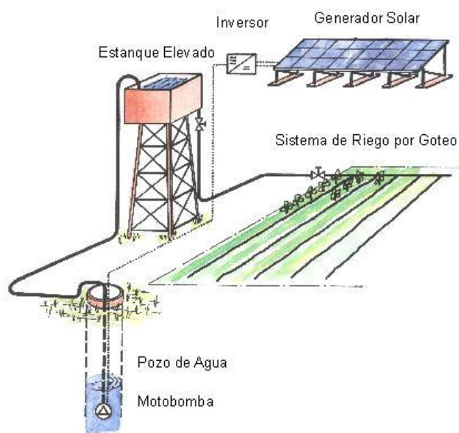
Figura 3.10. Sistema de riego Fotovoltaico
