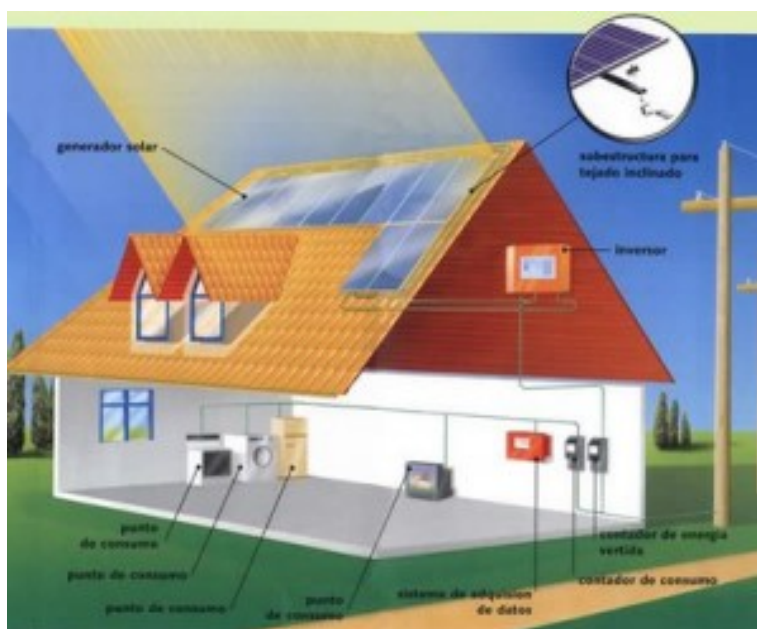
Figura 3.8. Instalación Fotovoltaica Alterna para viviendas
