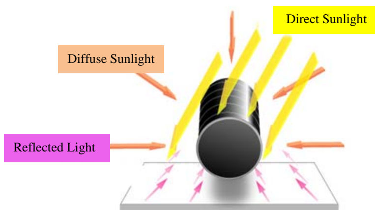
Figura 3.23. Absorción de luz de la célula cilíndrica
