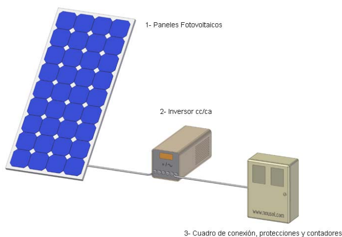
Figura 3.5. Sistema conectado a la red
