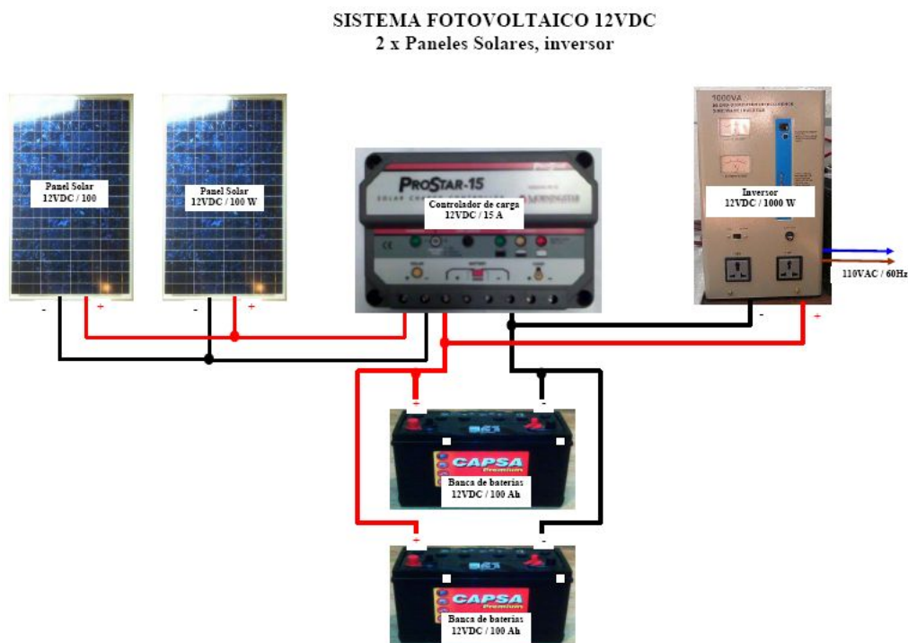
Figura 4.6. Sistema de Generación Fotovoltaica de 600Wh/día
