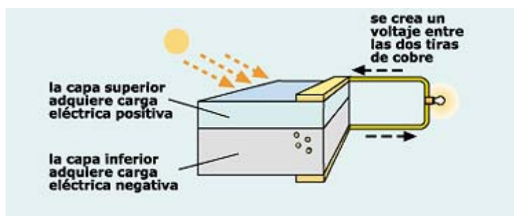
Figura 3.14c. A mayor nivel de de iluminación aumenta la entrega de energía
