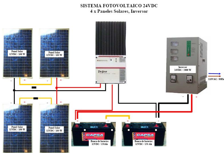
Figura 4.5. Sistema de Generación Fotovoltaica de 1.2kWh/día
