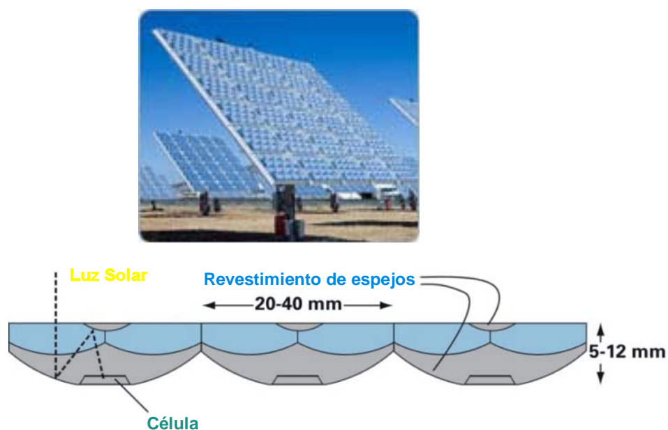
Figura 3.27. Sistema de captación y dirección de luz
