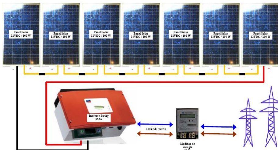
Figura 4.4. Sistema de Generación Fotovoltaica de 2.1kWh/día
