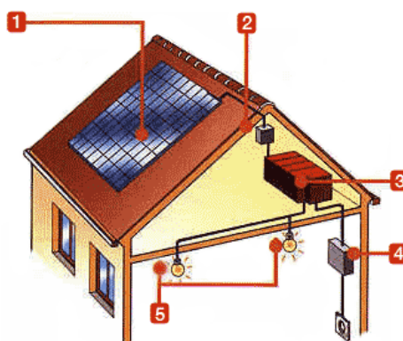
Figura 4.2. Instalación en una Vivienda
