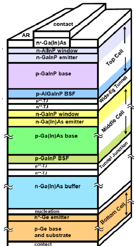
Figura 3.26. Composición de una célula de uniones múltiples
