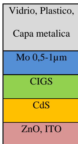
Figura 3.21. Estructura de una célula de CIGS
