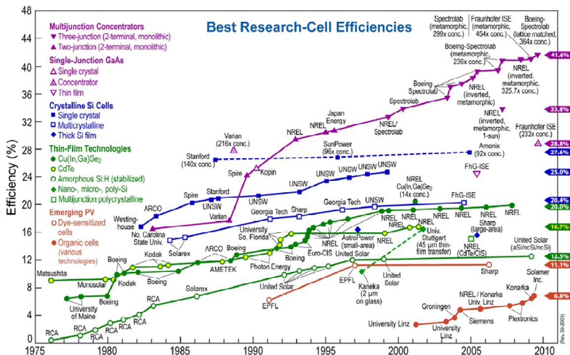
Figura 3.17. Evolución de la eficiencia con el tiempo y materiales
