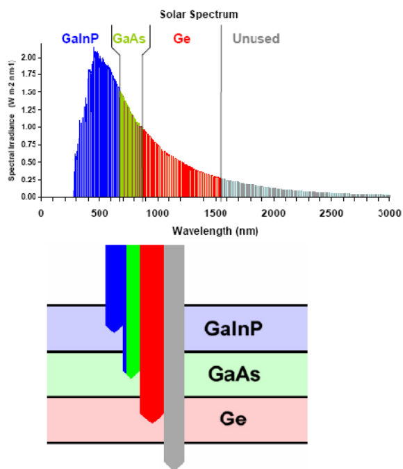
Figura 3.16. Distribución de las diferentes capas para alta eficiencia
