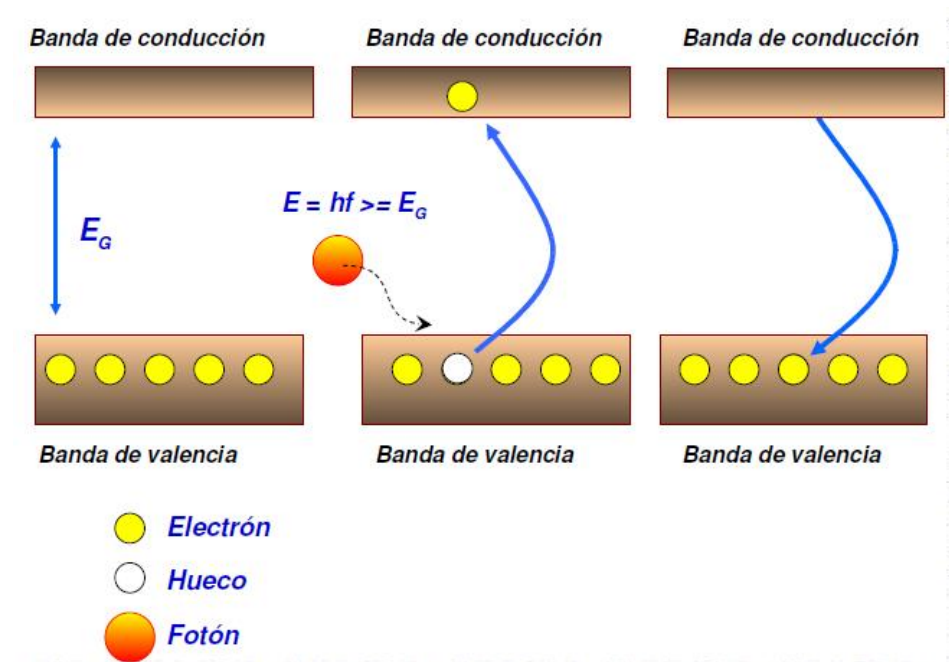
Figura 3.13. Proceso de Generación y Recombinación
