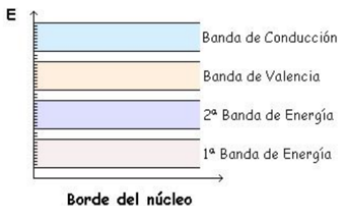
Figura 3.11. Distintas bandas energéticas de los cristales
