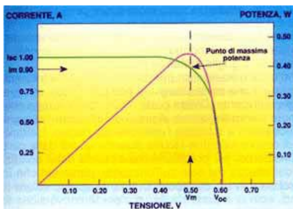
Figura 3.12b. Gráfica de Potencia de un Módulo Fotovoltaico
