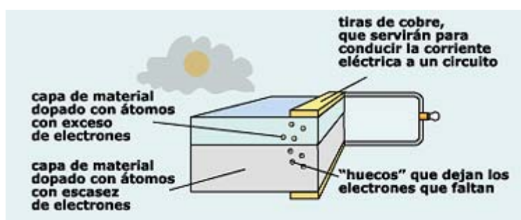
Figura 3.14a. Sistema en ausencia de luz solar
