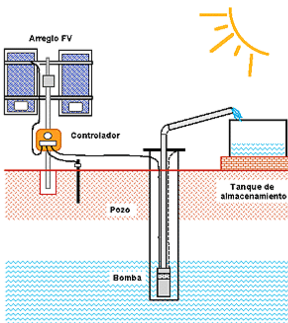
Figura 4.8. Configuración del Sistema Fotovoltaico para Bombeo de Agua
