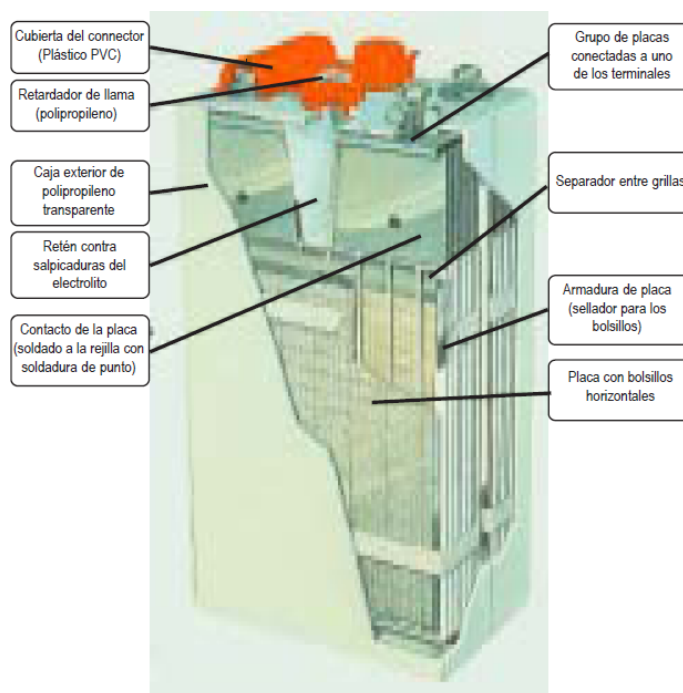
Figura 3.31. Batería de Níquel y Cadmio (SAFT-NIFE)
