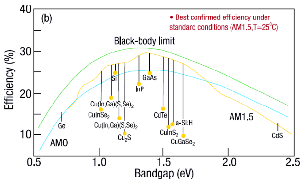
Figura 3.15. Relación de eficiencia vs. la banda gap. (Factores de voltaje y corriente)
