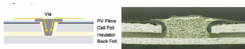
Figura 3.22a. Formación de células nanosolares
