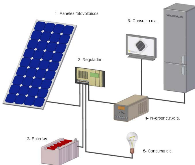
Figura 3.6. Sistema no conectado a la red
