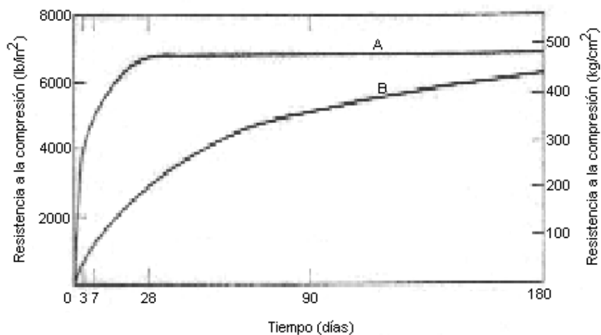
FIGURA 2.2. CURVAS DE RESISTENCIA A LA COMPRESIÓN FRENTE AL TIEMPO DE CURADO PARA MORTEROS PREPARADOS EN RELACIÓN 1:3 CON DOS CEMENTOS PÓRTLAND DIFERENTES A=70% C_3S , 10% C_2S . B=30% C_3S , 50% C_2S . [7]
