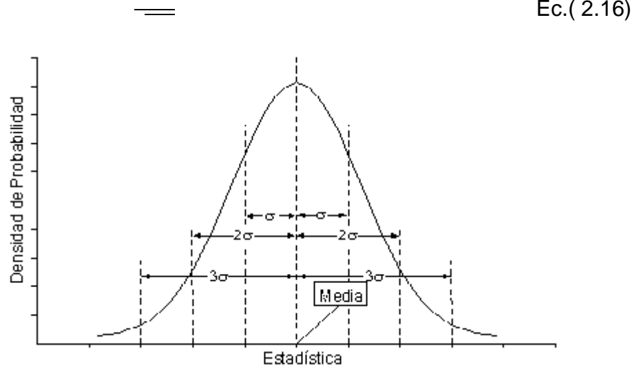
FIGURA 2.8. GRÁFICA DE LA DENSIDAD DE PROBABILIDAD NORMAL [16].
