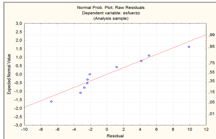
FIGURA 4.6. GRÁFICA DE PROBABILIDAD NORMAL DE LOS RESIDUOS PARA PASTAS DE CEMENTO CON 20% DE LIMOLITA.
