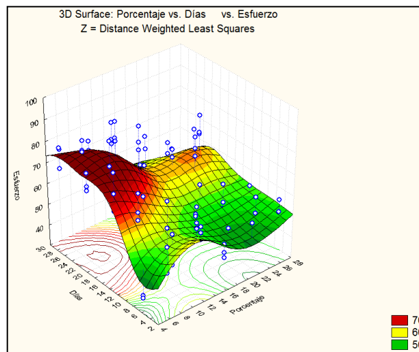
FIGURA 4.16. SUPERFICIE DE RESPUESTA PARA DÍAS DE CURADO Y PORCENTAJE DE LIMOLITA
