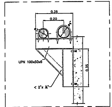
DETALLE DE SOPORTE DE PARED
