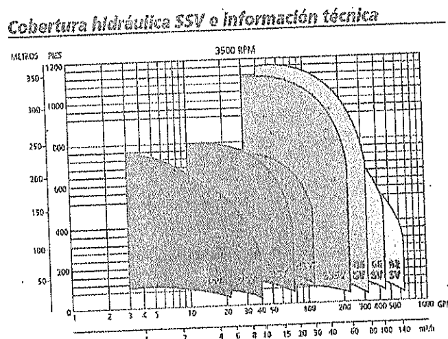
FIGURA 3.4.a. COBERTURA HIDRAULICA DE BOMBAS MULTIETAPAS VERTICALES
