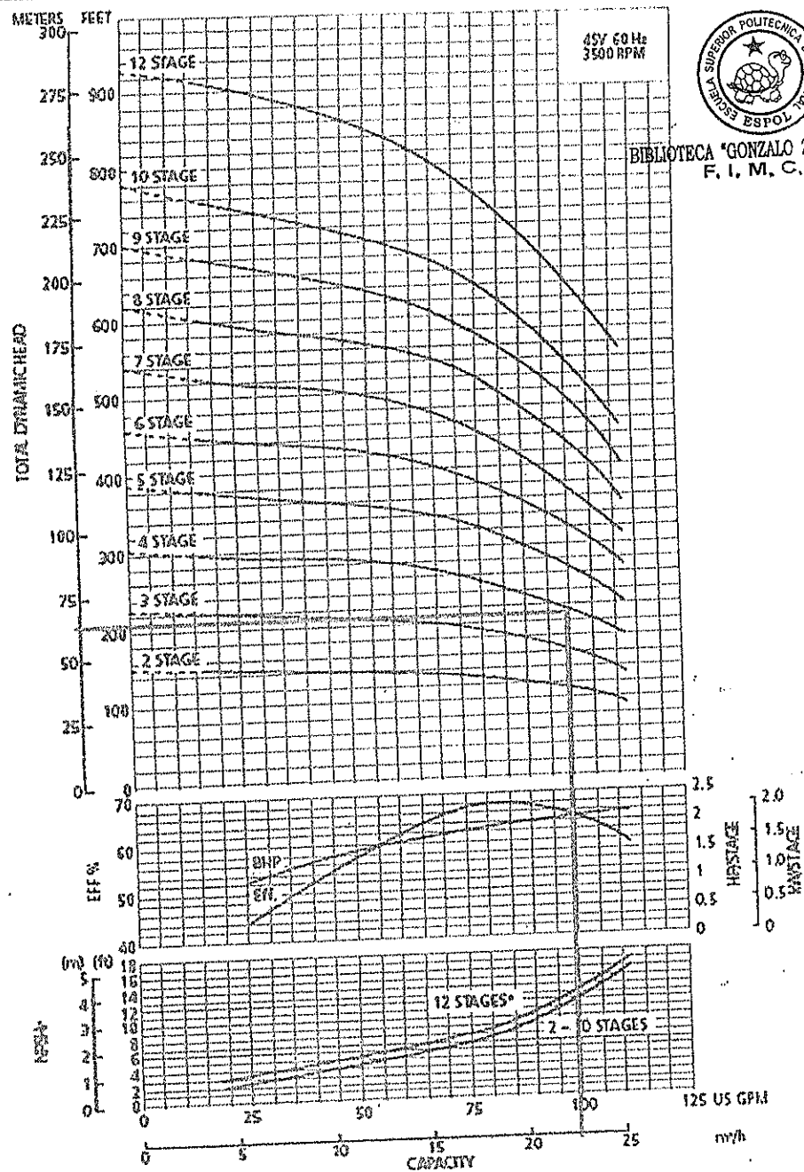
FIGURA 3.5.b. CURVA HIDRAULICA PARA BOMBAS 4SV
