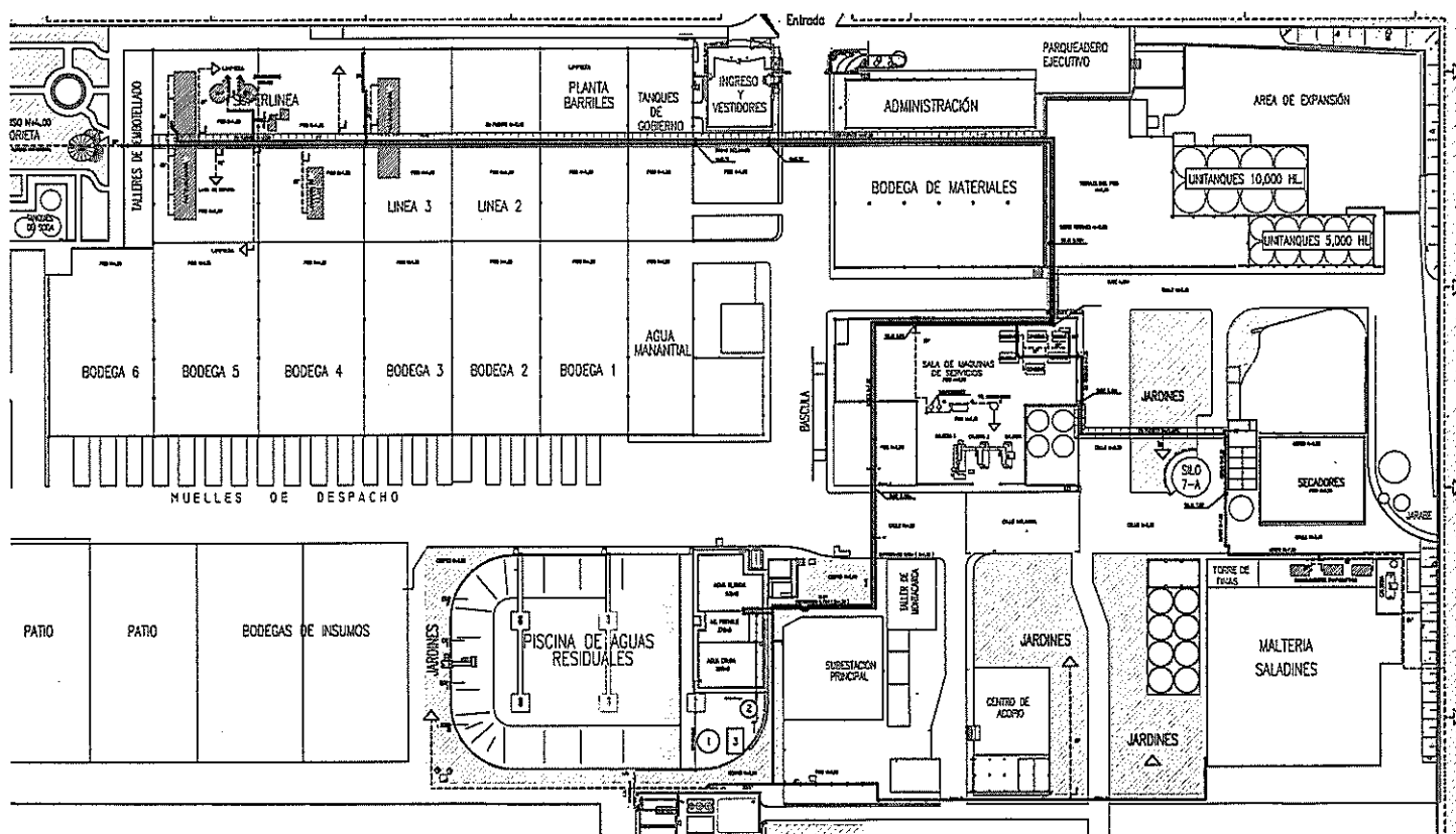
VISTA DE PLANTA ESCALA 1:750
