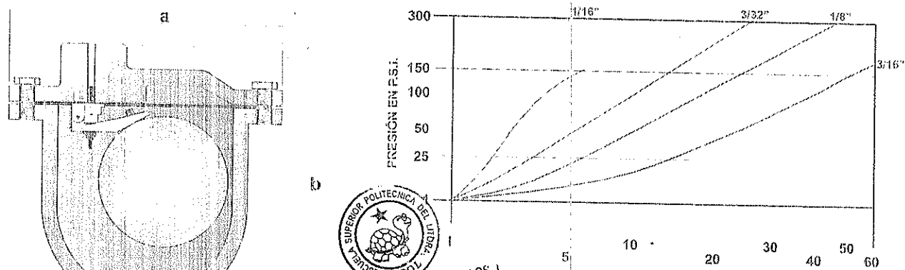
CAPACIDAD DE VENTEO SEGÚN PRESIÓN DE TRABAJO Y DIÁMETRO DE ORIFICIO DE VENTEO
