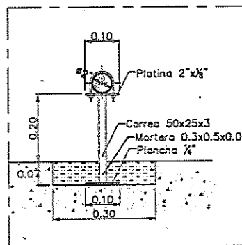
DETALLE "8"
