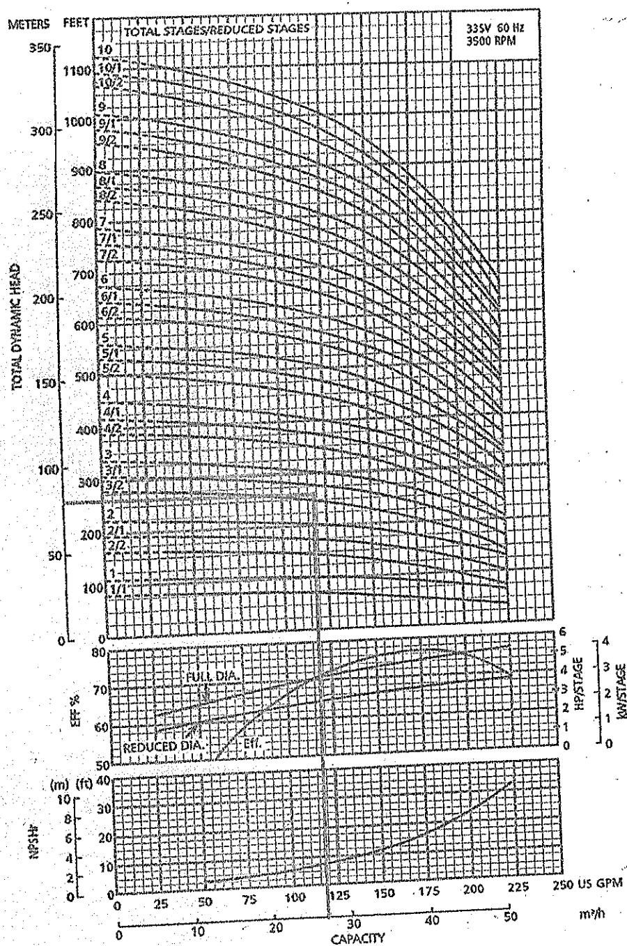
FIGURA 3.4.d. CURVA HIDRAULICA PARA BOMBAS 33SV
