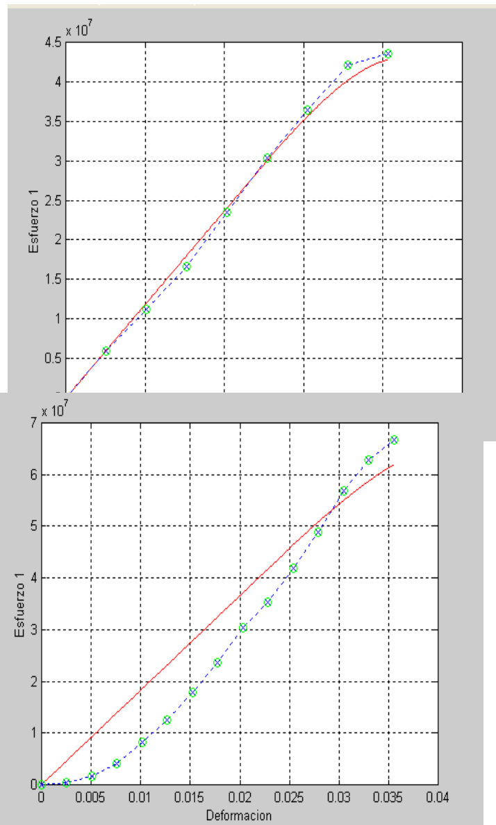
FIGURA 4.25 VALIDACIÓN DEL MODELO A LOS 7 DÍAS
