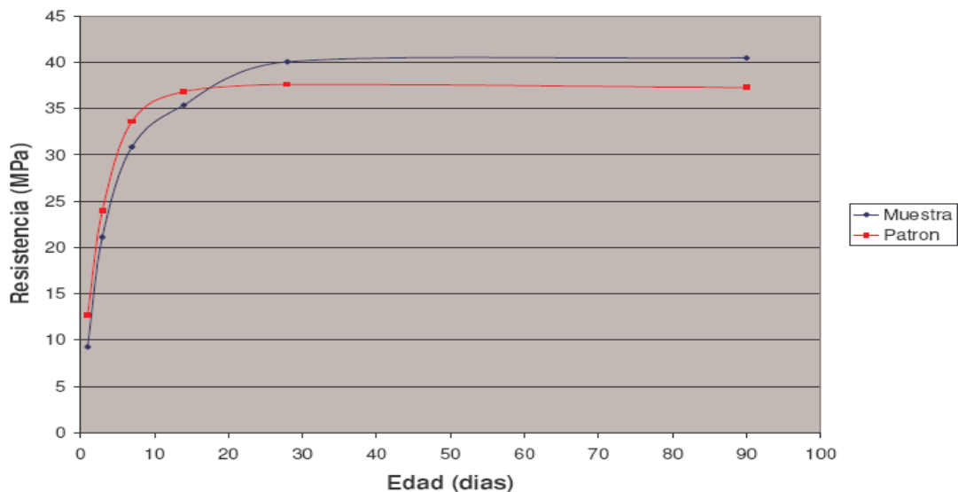
FIG 2.9 COMPARACION DE RESISTENCIAS MUESTRA/PATRON
