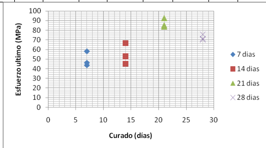
FIGURA 4.9 GRÁFICA ESFUERZO ÚLTIMO VS. CURADO – 10% DE LIMOLITA
