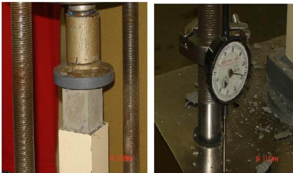
FIG 3.11 ENSAYO DE COMPRESIÓN
