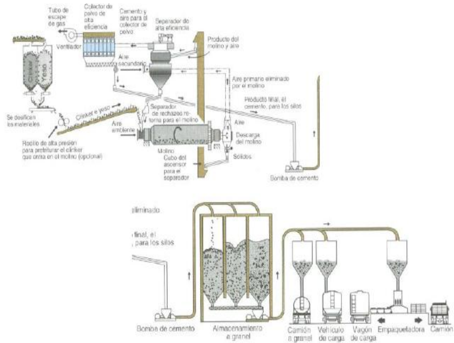
FIG 2.4 MOLIENDA
