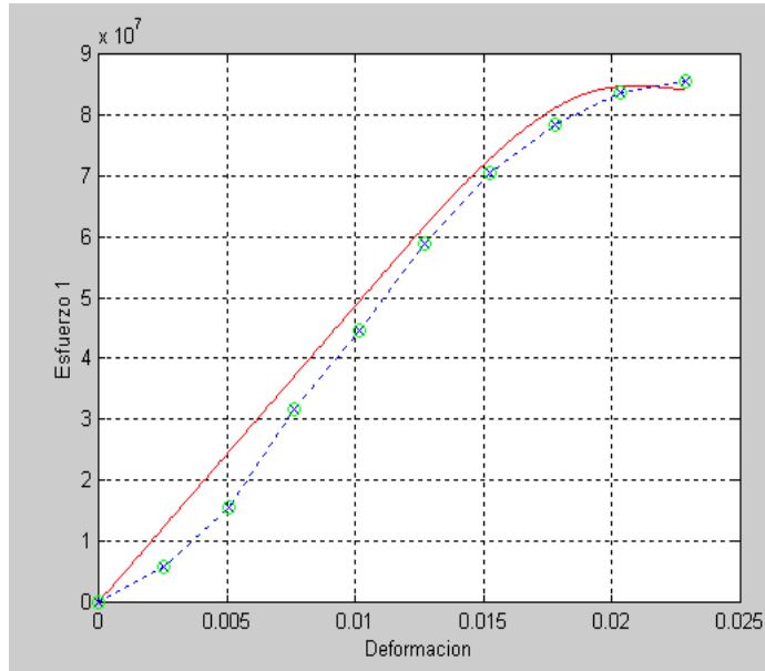
FIGURA 4.27 VALIDACIÓN DEL MODELO A LOS 21 DÍAS
