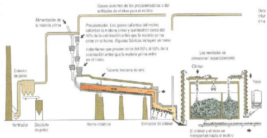
FIG 2.3 CALCINACION
