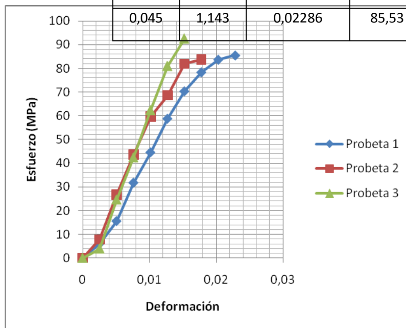
FIGURA 4.3 GRAFICA ESFUERZO – DEFORMACIÓN (G3/10/21)
