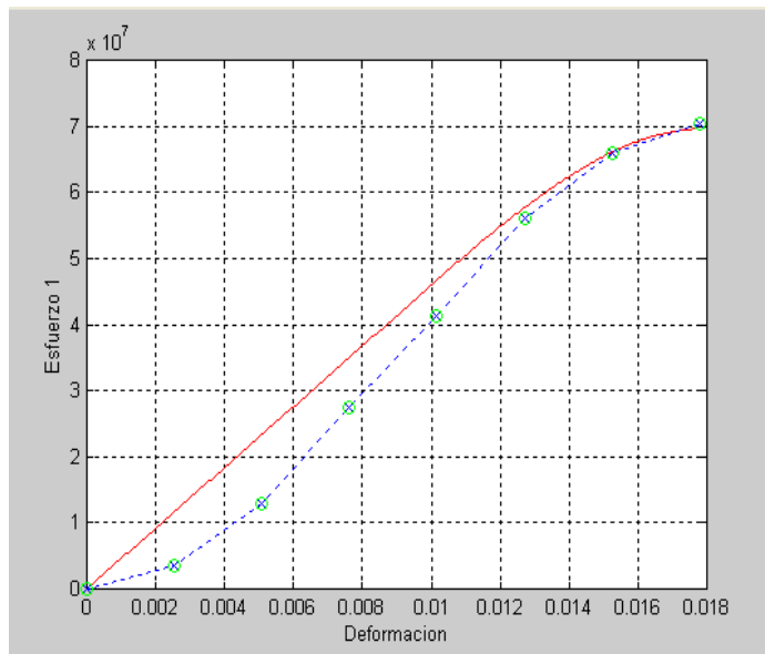
FIGURA 4.28 VALIDACIÓN DEL MODELO A LOS 28 DÍAS
