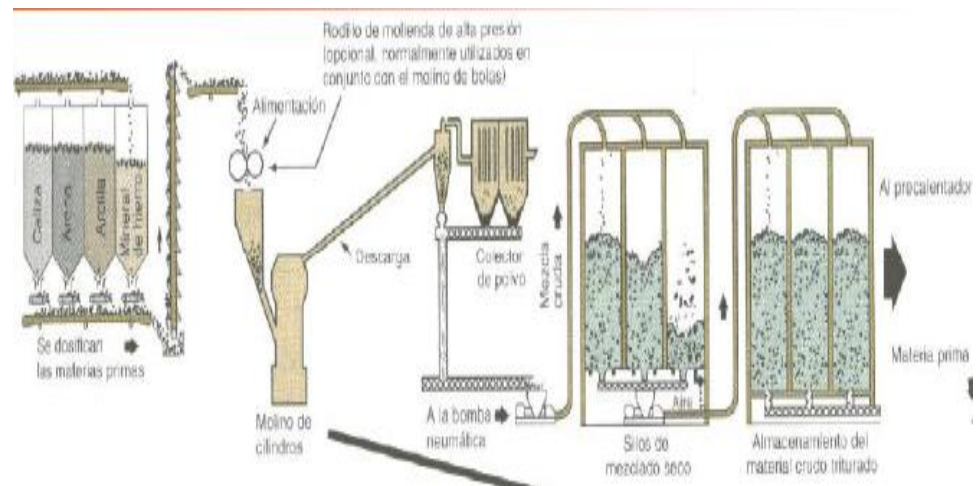
FIG 2.2 MOLIENDA Y HOMOGENIZACION Fuente: Carrasco Fernanda, Materiales Cementicios, 2007
