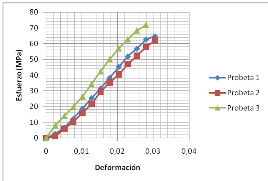
FIGURA 4.5 GRAFICA ESFUERZO – DEFORMACIÓN (G3/12.5/4)
