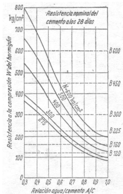
FIG 2.8 RESISTENCIA A LA COMPRESION DEL HORMIGON EN FUNCIÓN DE A/C
