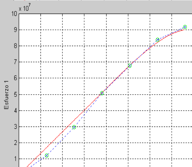
FIGURA 4.31 VALIDACIÓN DEL MODELO A LOS 18 DÍAS
