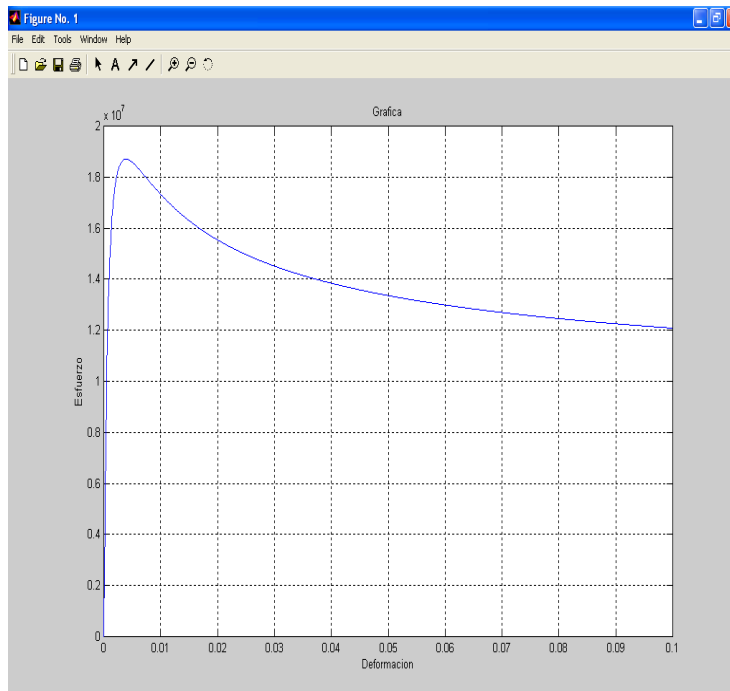
FIG.3.14 GRAFICA ESFUERZO Vs. DEFORMACIÓN (MODELO MATEMATICO)
