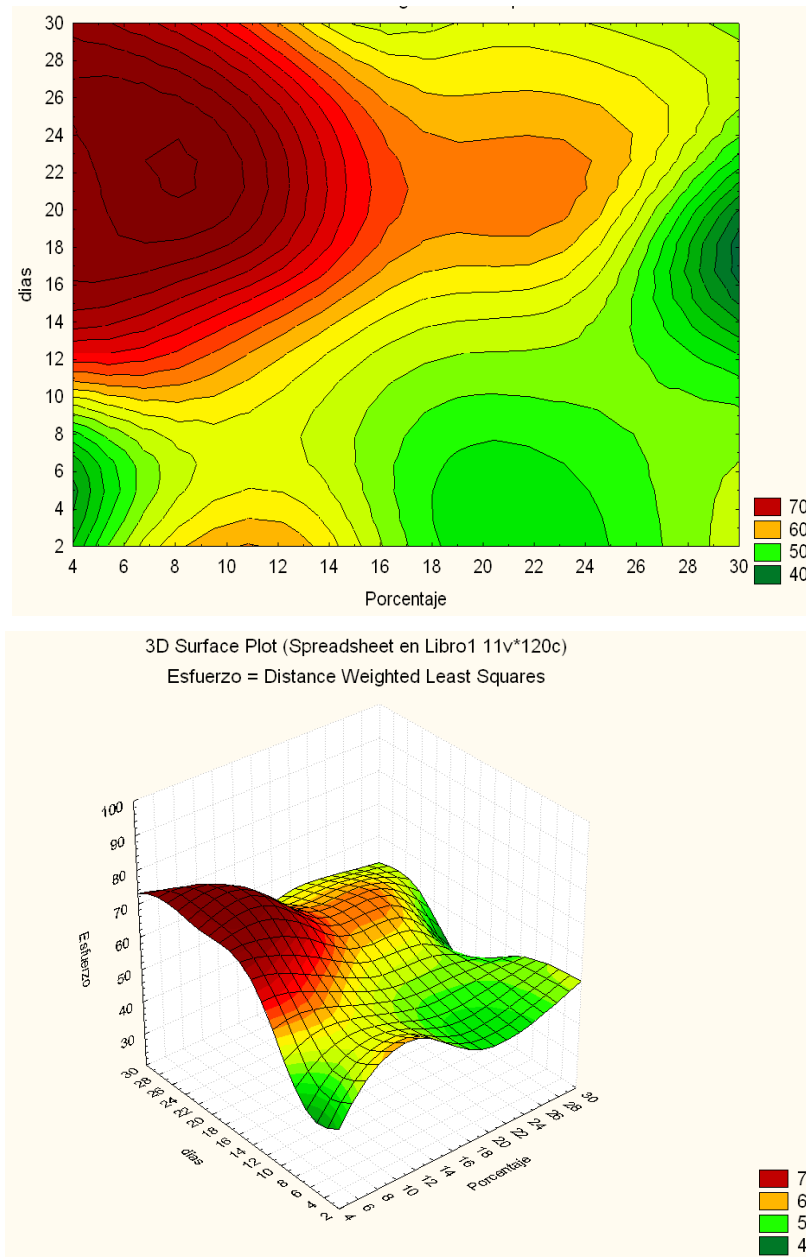
FIGURA 4.24 GRÁFICA GLOBAL DE ESFUERZOS ÚLTIMOS, DÍAS Y PORCENTAJES
