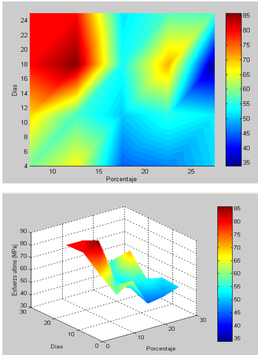
FIGURA 4.23 GRÁFICA DE ESFUERZOS ÚLTIMOS, DÍAS Y PORCENTAJES DE ADITIVOS (VALIDACIÓN)
