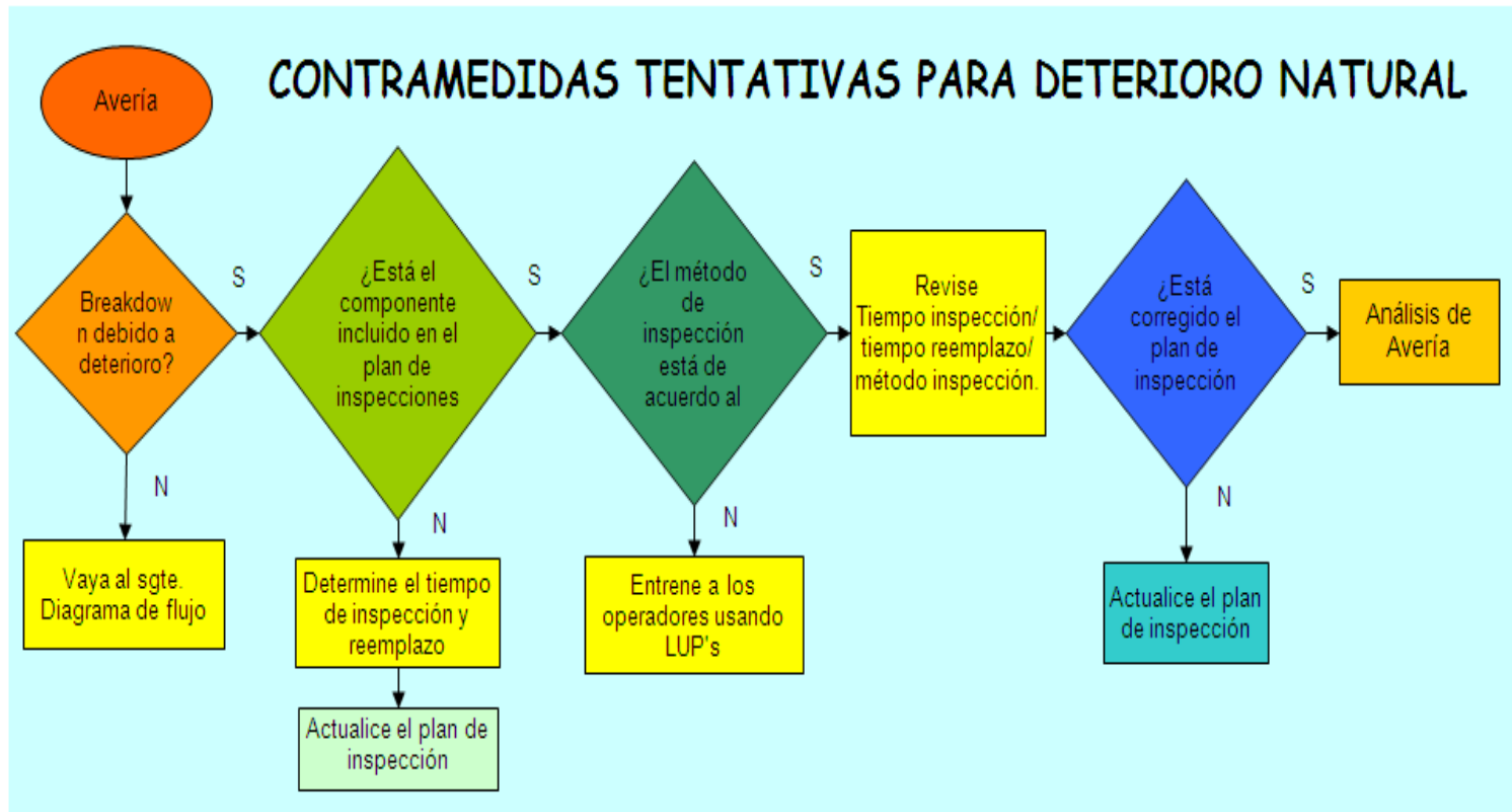
FIGURA 3.9: FLUJO PARA LA CONTRAMEDIDA PUNTO DÉBIL DE DISEÑO
