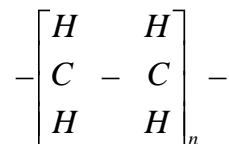
FIGURA 2.3 ESTRUCTURA QUÍMICA DEL ETENO (ETILENO)
