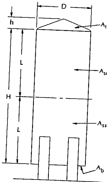
Fig. 3a – Areas de Diseño para Tanques Verticales
