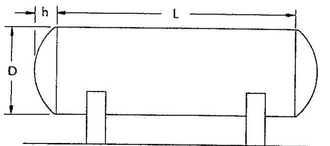
Fig. 1a – Áreas de Diseño para Tanques Horizontales
