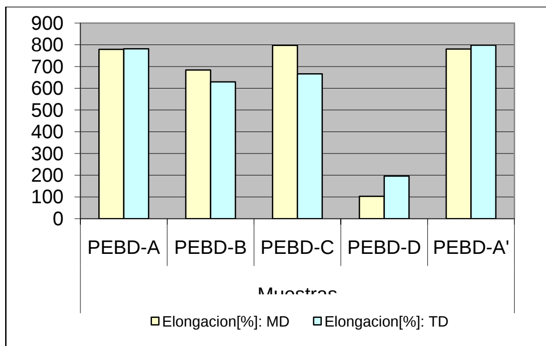
FIGURA 4.7 ELONGACIÓN MD Y TD
