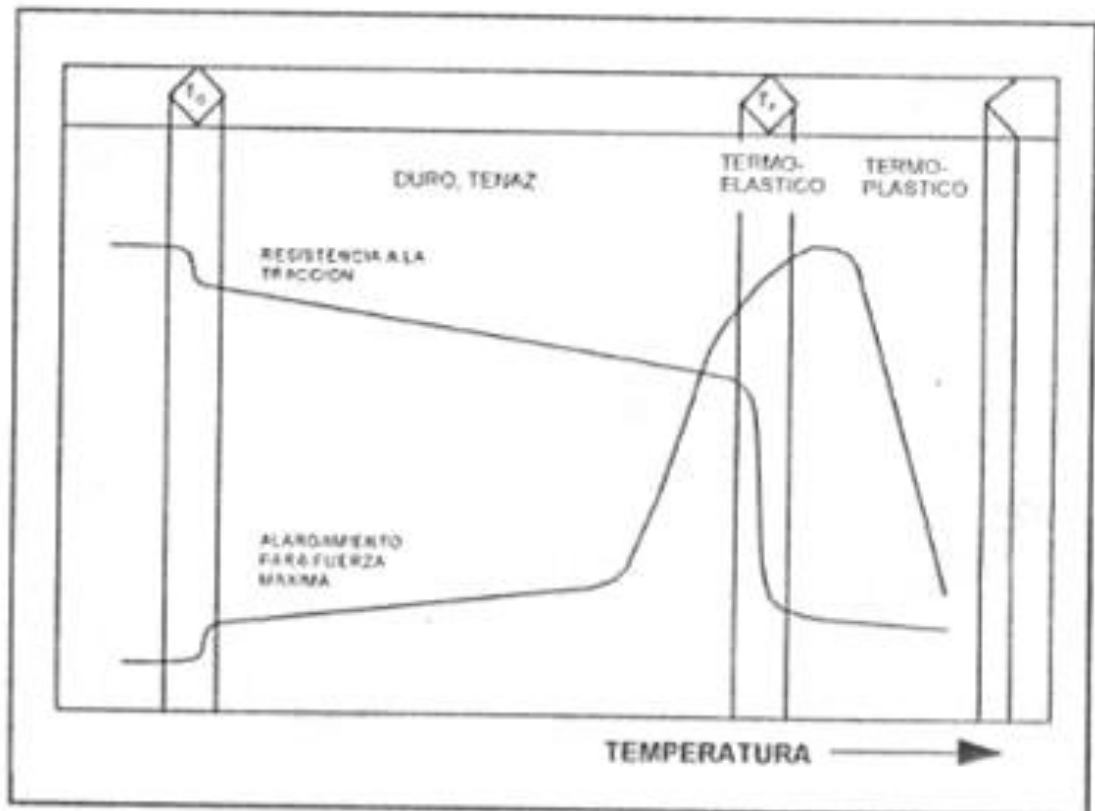
DIAGRAMA DE ESTADO DE LOS TERMOPLÁSTICOS CRISTALINOS
