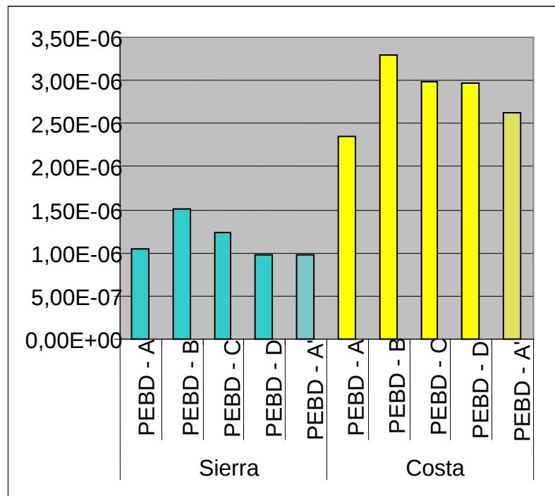
FIGURA 4.19 TASA DE TRANSFERENCIA DE VAPOR DE AGUA
