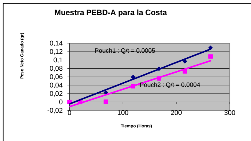
FIGURA 4.13 CURVA Q/T PARA PEBD-A A CONDICIONES DE LA COSTA
