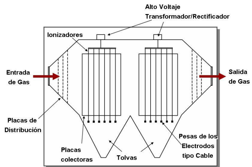
FIGURA 2.3. PRECIPITADOR ELECTROSTÁTICO
