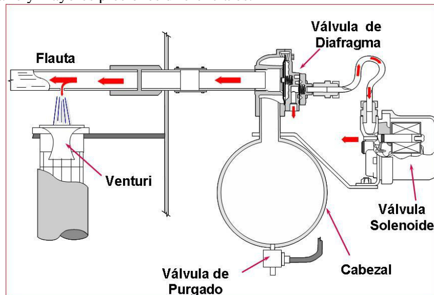
FIGURA 3.39. Limpieza por aire comprimido para pulse-jet. Es esencial para una buena operación del sistema, libre de problemas, que la calidad del aire comprimido sea buena, es decir que este sea seco, además de un buen volumen de aire. Usualmente la presión requerida para la limpieza es de 6 bar.
