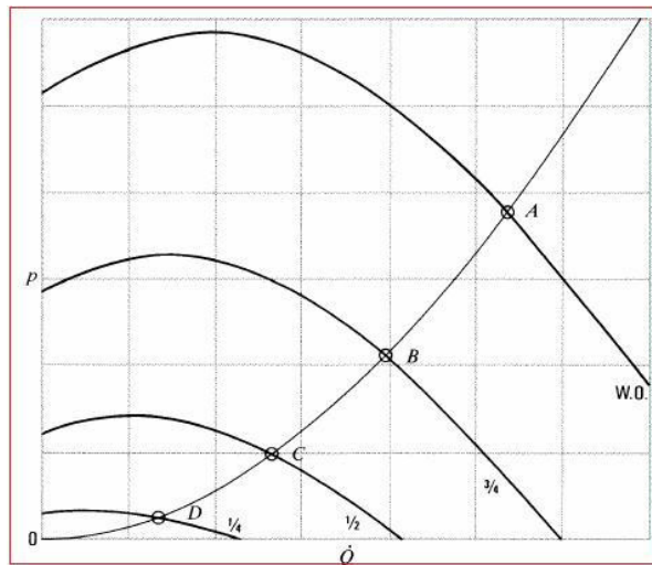
FIGURA 3.38. Operación con velocidad variable
