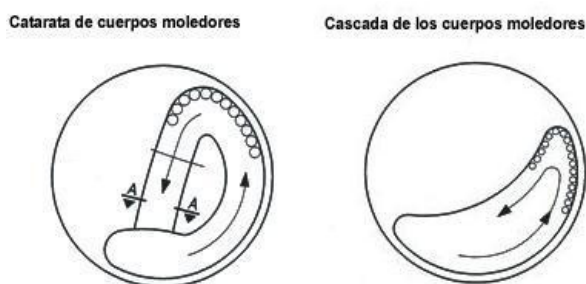
FIGURA 1.8. Efecto de los cuerpos molidores en un molino tubular
