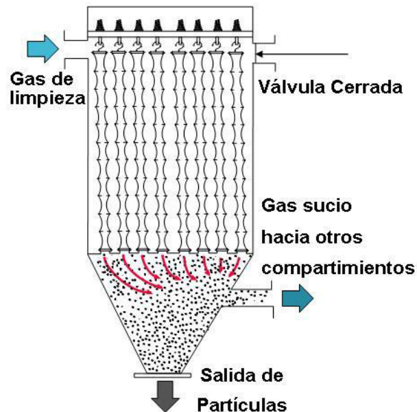
FIGURA 2.8. FILTRADO INTERIOR
