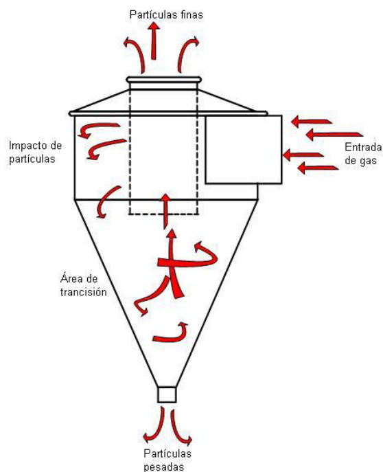
FIGURA 2.1. CICLÓN
