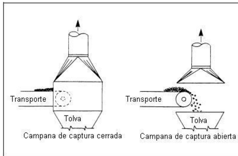
FIGURA 3.3. Tipos de campanas de captura
