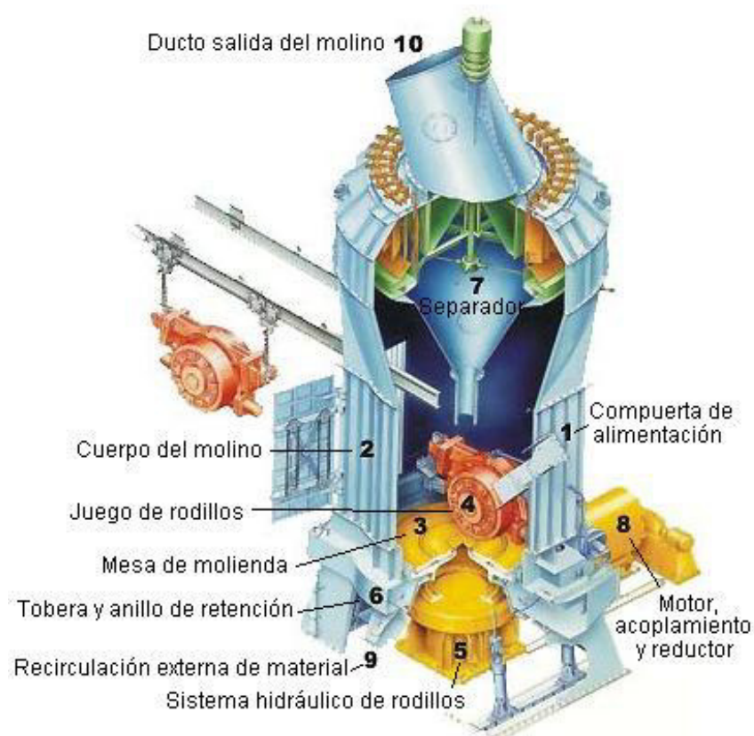
FIGURA 1.6. Molino vertical
