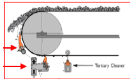
FIGURA 4.9. CEPILLOS DE LIMPIEZA PRIMARIO, SECUNDARIO Y Terciario
