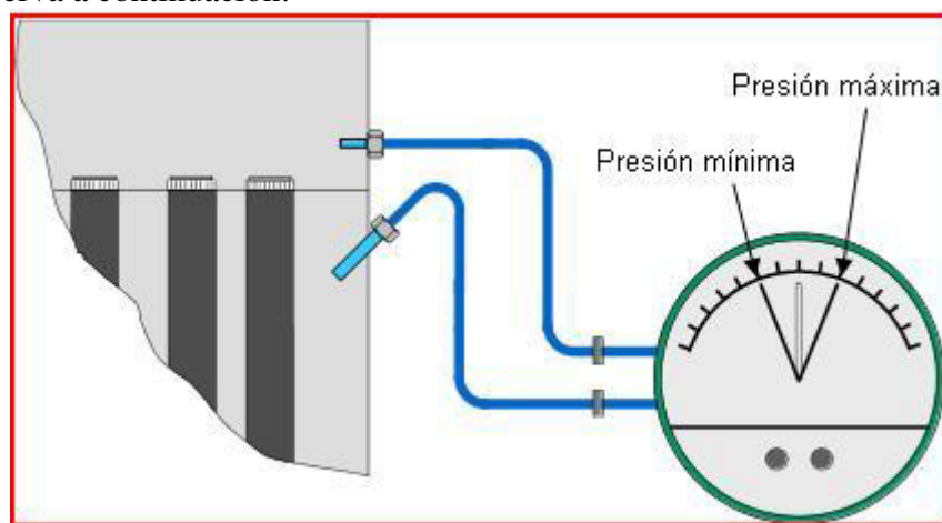
FIGURA 3.41. Manómetro diferencial.
