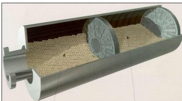
FIGURA 1.9. Molino tubular
