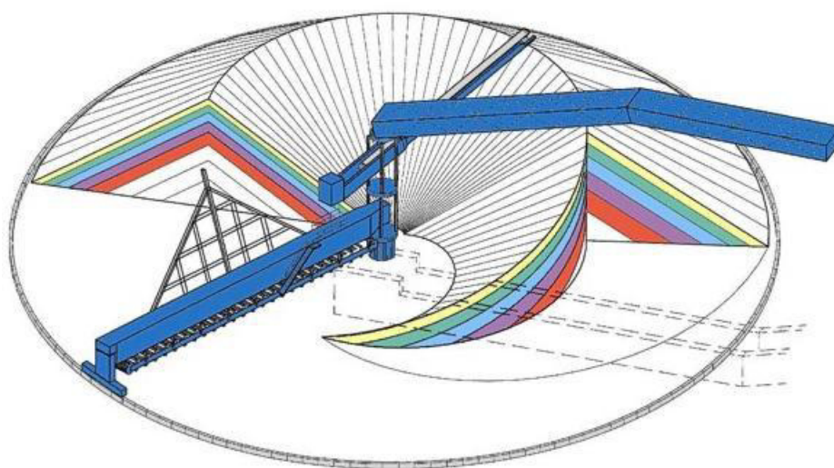
FIGURA 1.4. Apilamiento y prehomogenización del material
