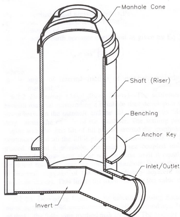
Figura 1.4 Partes de cámaras de inspección y manholes.
