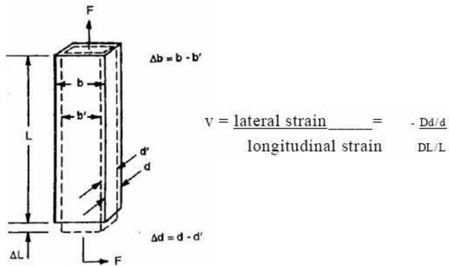
Figura 2.3 Una barra en tensión muestra los cambios dimensionales.
