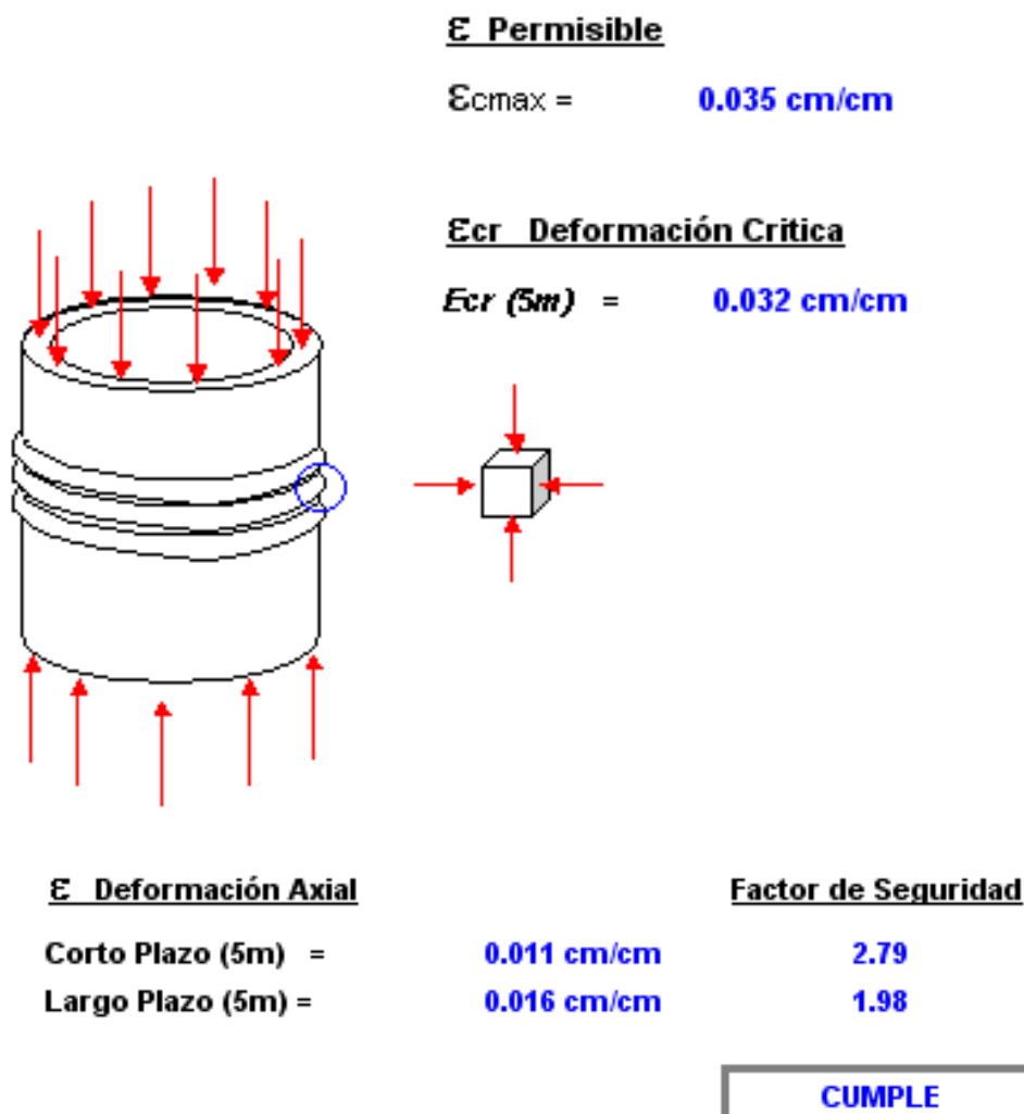
Figura 4.8 Resumen de análisis de Compresión y Pandeo axial.
