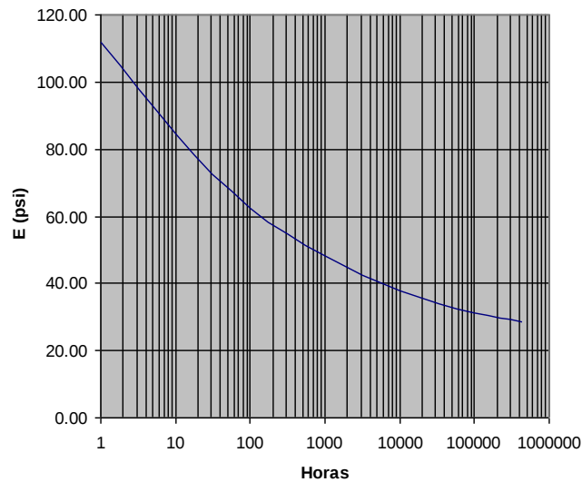
Figura 4.2 Curva de modulo de Relajación vs tiempo para HDPE
