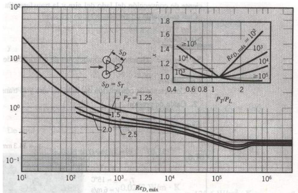
Figura 4.7 Curva para determinar el factor de fricción para arreglo de tubos escalonados.
