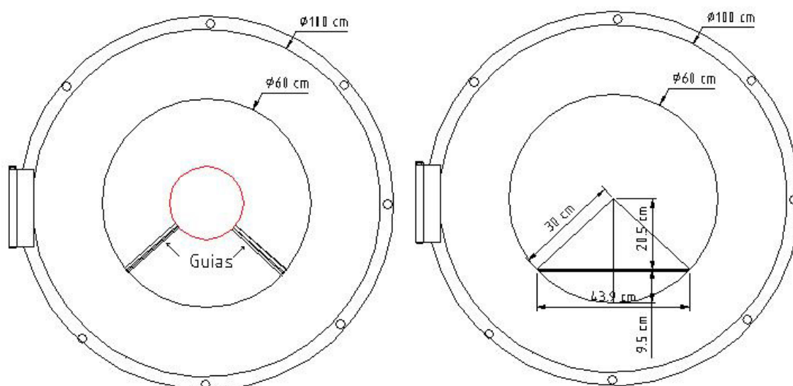
Figura 3.9 Esquema de la localización de las Guías y de la parrilla en el interior de la primera cámara
