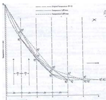
Figura 3.2 Gráfico del Método de Schmidt
