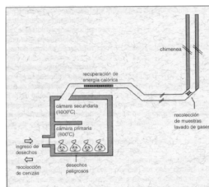
Figura 2.1. Incinerador de dos cámaras
