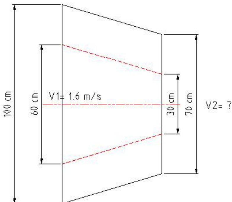
Figura 4.3 Dimensionamiento del acople
