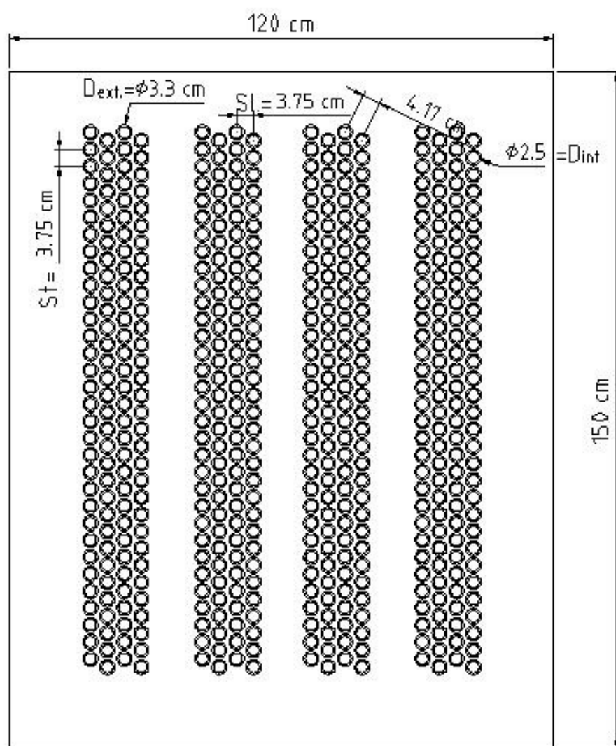
Figura 4.8 Esquema del Intercambiador.
