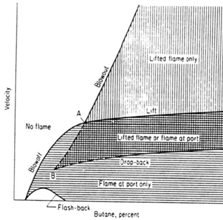
Figura 3.12 Soplando de quemadores
