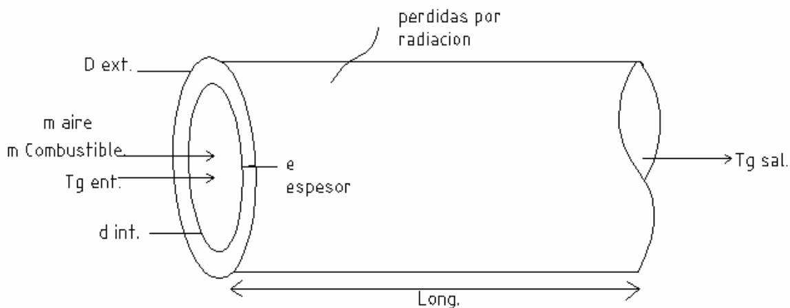
Figura 3.7 Flujos de entradas y salidas en el proceso
