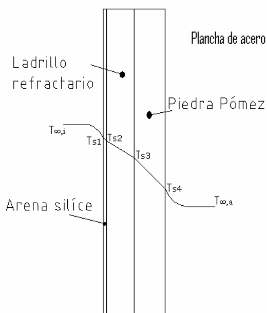
Figura 3.1 Esquema de la pared del incinerador
