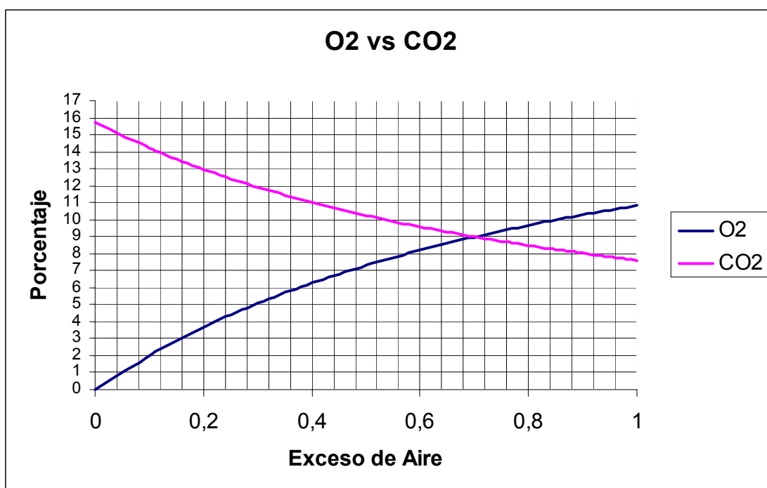
Figura 4.2 Diagrama de Ostwald
