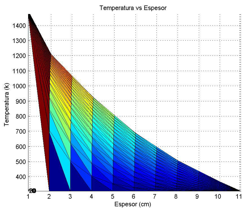
Figura 3.4 Grafica de superficie en base al método de Schmidt
