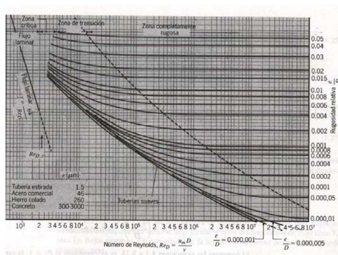
Figura 4.12 Factor de fricción para flujo completamente desarrollado en un tubo circular
