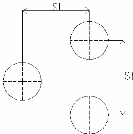
Figura 4.5 . Arreglos de tubos en un banco de tubo escalonado
