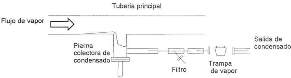
Figura 5.3. Conjunto trampa de vapor
