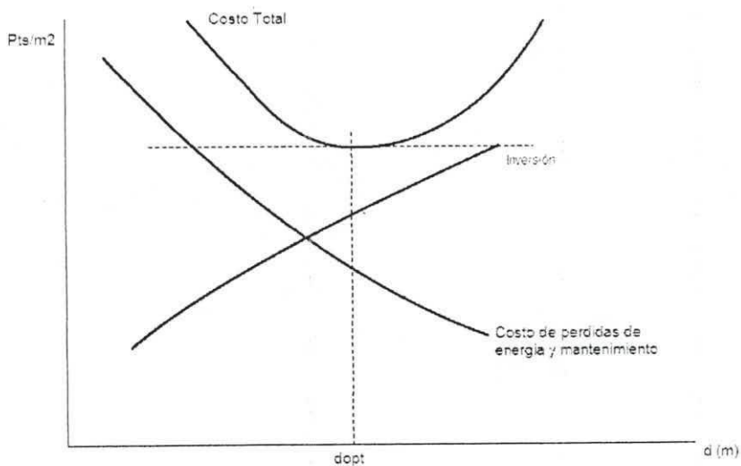
Figura 5.2. Espesor óptimo económico de aislamiento térmico
