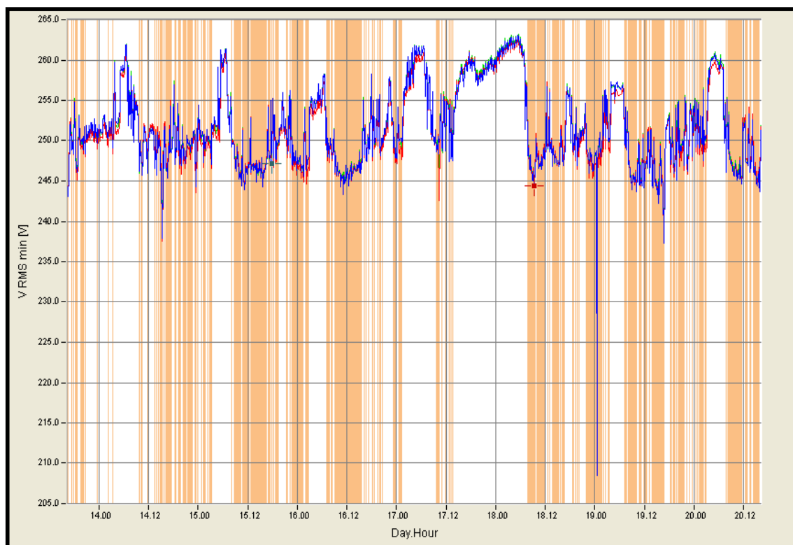
Figura 5.3 Espectro de Voltaje mínimos Enero 2010 BLOQCIM S.A.
