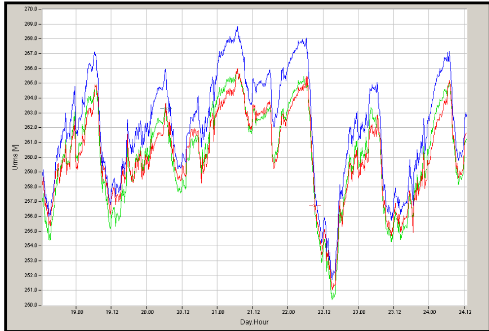
Figura 5.14. Espectro de Voltajes medios de la medición Diciembre 2008
