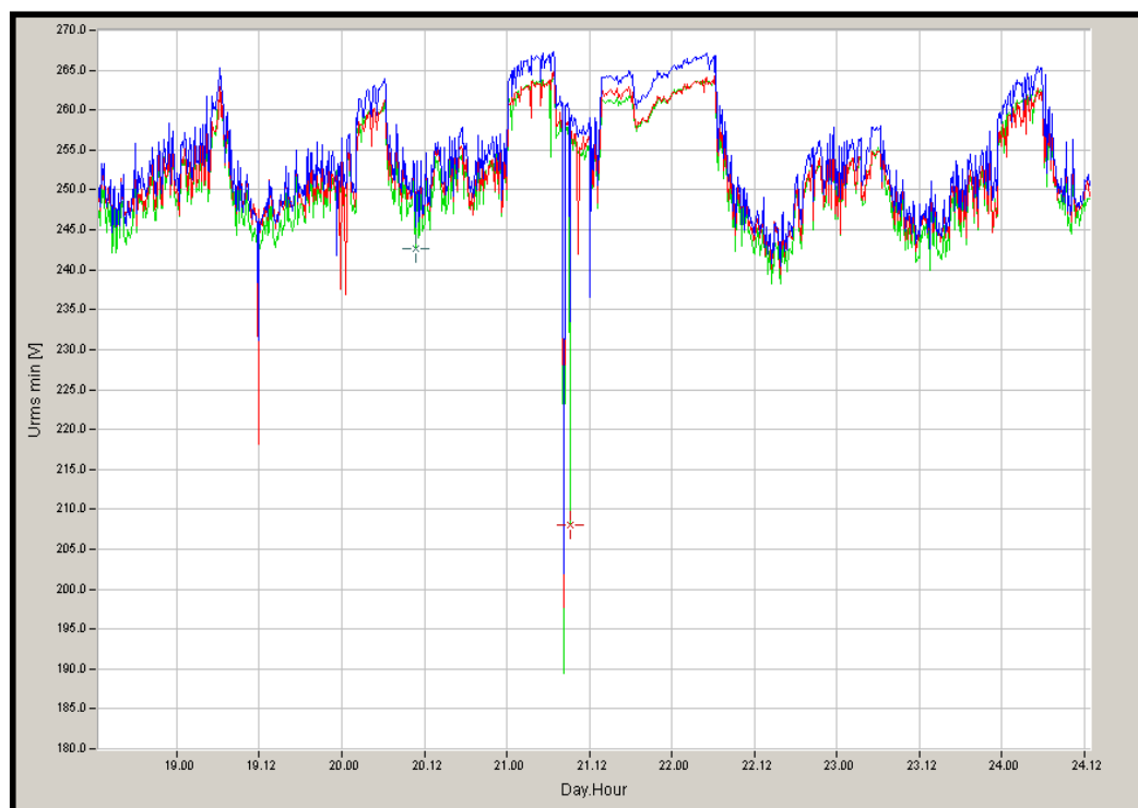
Figura 5.1 Espectro de Voltaje mínimos Diciembre 2008 BLOQCIM S.A.
