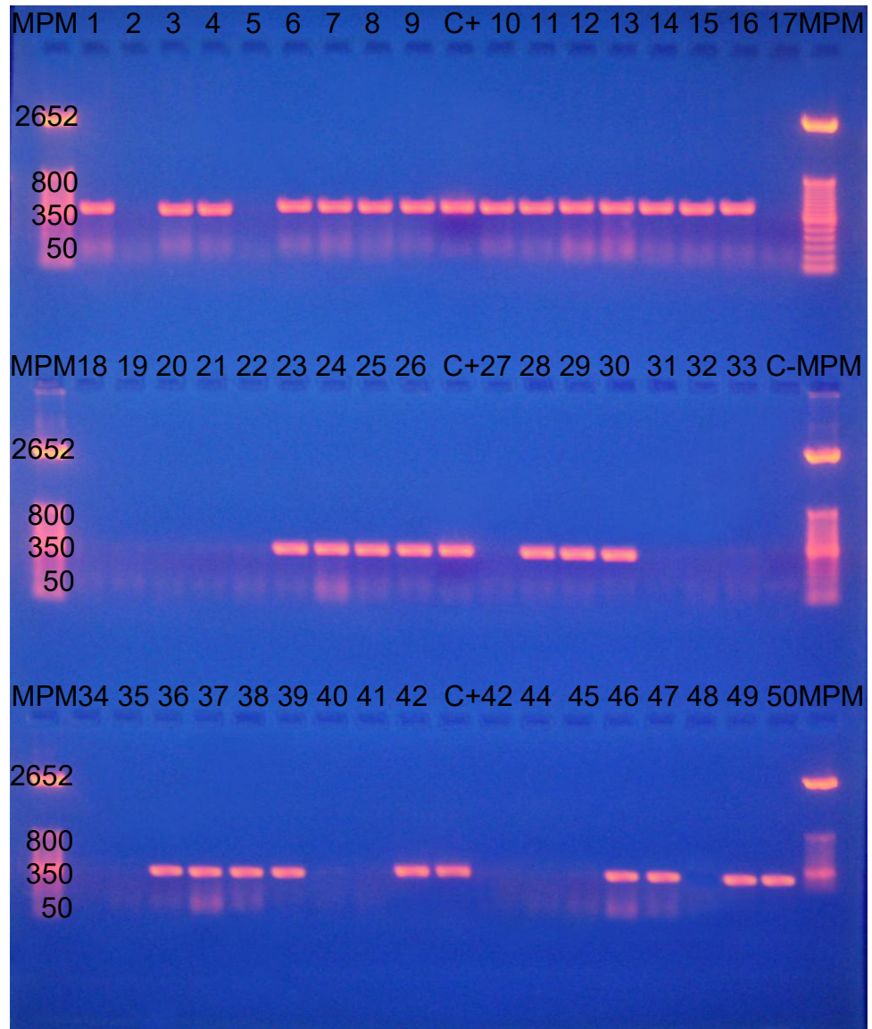
Foto 8. Reacciones de amplificación de PCR reveladas en geles de agarosa 1,2% para la detección de IHHNV Lote B-21, Post - larva 14, B2. 1-50: Reacciones de PCR. MPM = Marcador de peso molecular; C+ = Control positivo banda de 345pb. C- = Control negativo (Fuente: R. Marcillo Del C. Ayangue 2.009).
