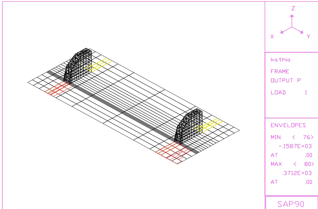
Figura 3.15 Máximas fuerzas generadas en los ángulos
