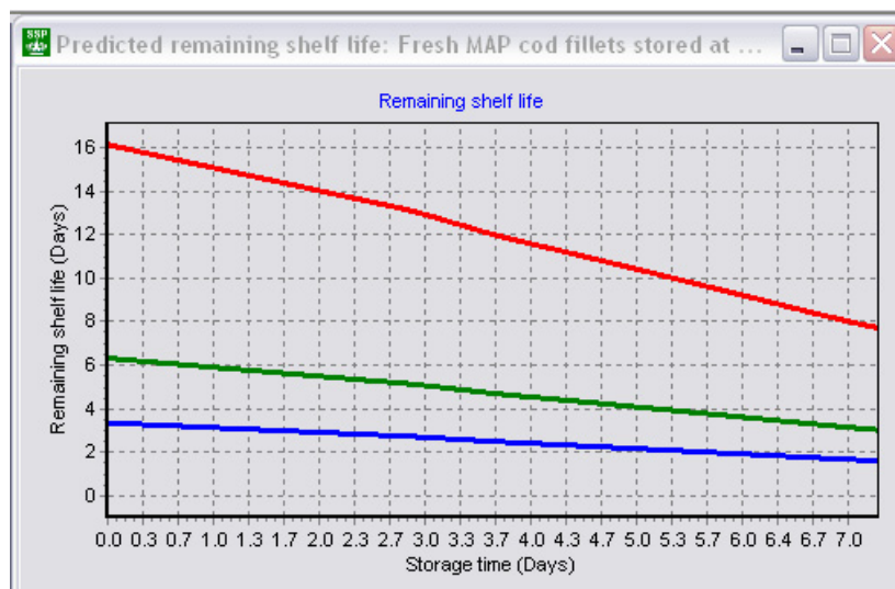
Figura 3.2.2.3 Curva de reducción de vida útil.
