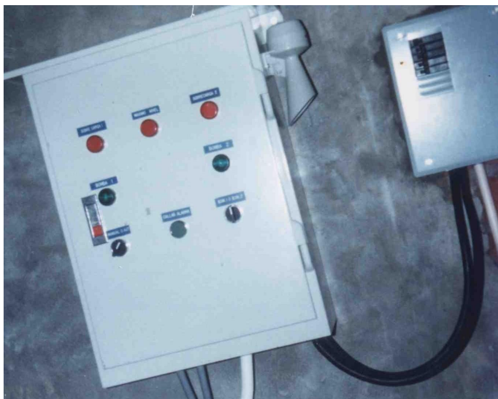
FIGURA 2.7 TABLERO DE CONTROL DE BOMBAS SUMERGIBLES
