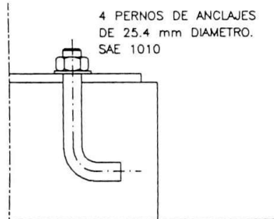
DETALLE N-N1 SIN ESCALA
