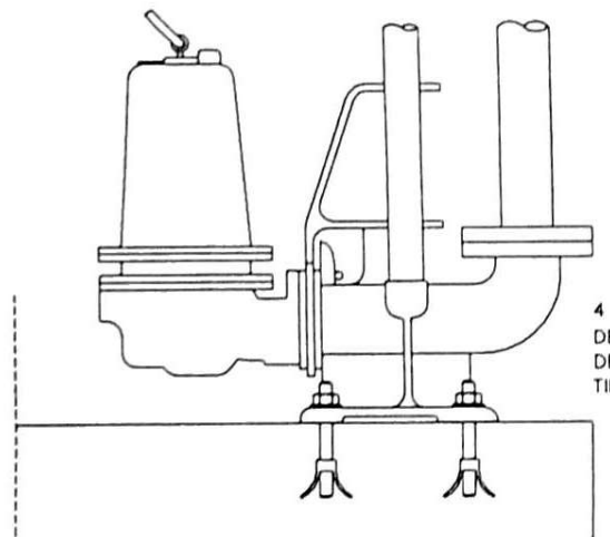
DETALLE R-R1 SIN ESCALA
