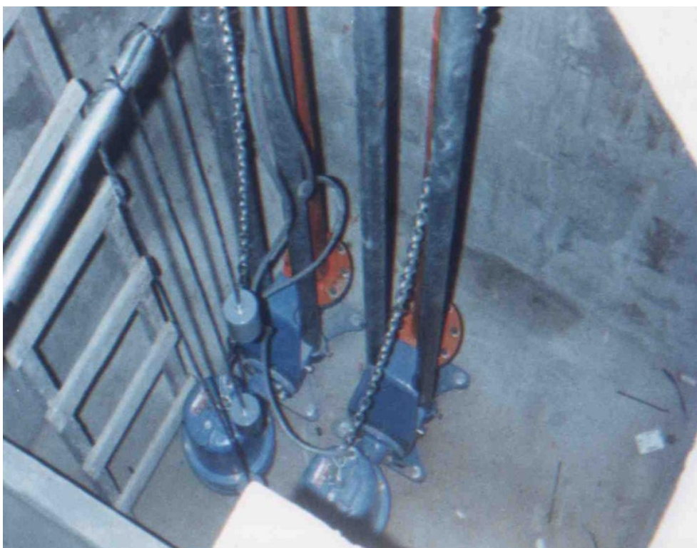
FIGURA 2.5: MONTAJE DE BOMBAS SUMERGIBLES
