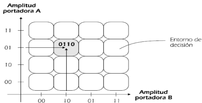
Fig.A.8. 16QAM
