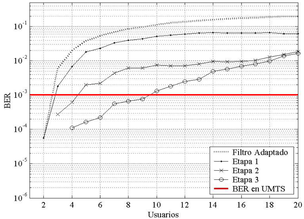
Fig.3.15.P-PIC 3 Etapas vs Número de usuarios con control de potencia perfecto. [27]
