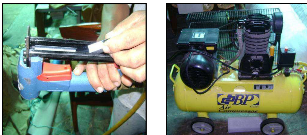
FIGURA 3.1 GRAPADORAS DE TACHUELAS Y GRAPAS
