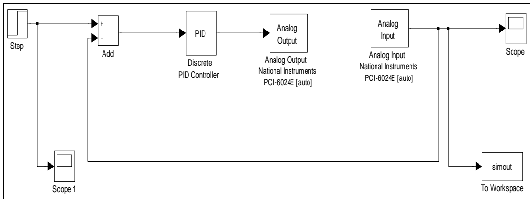
Figura 64 Diagrama de bloque de Simulink con el controlador planta real
