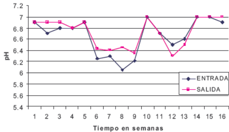
Figura 2.2 Evolución del pH en el interior y en el efluente de un biodigestor que trabaja con excretas de cerdo destinado para la producción de biogás (Romero y Simanca, 2005). Se observa tanto en el caldo (entrada) como el efluente (salida) inician el proceso con un pH cercano a 7, en las semanas 8 y 9 el pH baja entre 6 a 5.5, en adelante el pH sube y se mantiene alto en el caldo y el efluente.
