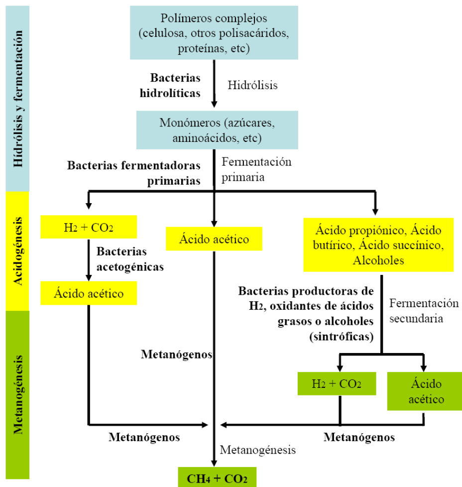
Figura 2.1 Esquema del proceso de producción de metano en fermentaciones anaeróbicas (Señer, 2005, adaptado por Robalino, 2010). El proceso se inicia a partir de polímeros complejos que son hidrolizados y fermentados hasta ácidos orgánicos varios, ácido acético, H_2 y CO_2 . Luego por fermentaciones secundarias y acetogénesis se obtiene ácido acético que finalmente por acción de los metanógenos forma metano y CO_2 al igual que el H_2 y CO_2 generado en las fermentaciones primaria y secundaria
