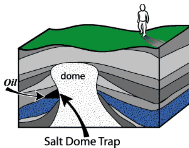
FIGURA 1.7 DOMO SALINO
