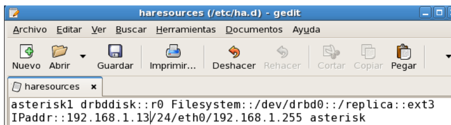
Fig. 9 Archivo /etc/ha.d/haresources
