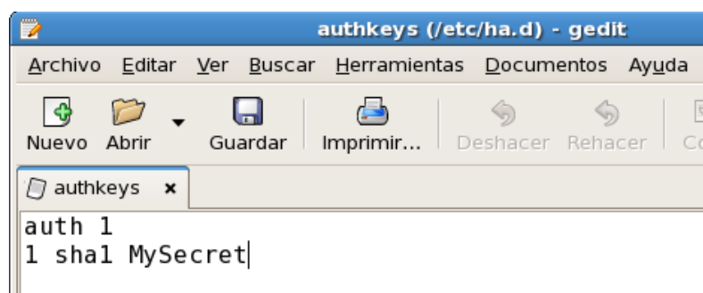
Fig. 8 Archivo /etc/ha.d/authkeys
