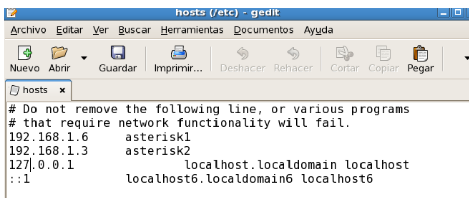
Fig. 3 Archivo /etc/hosts
