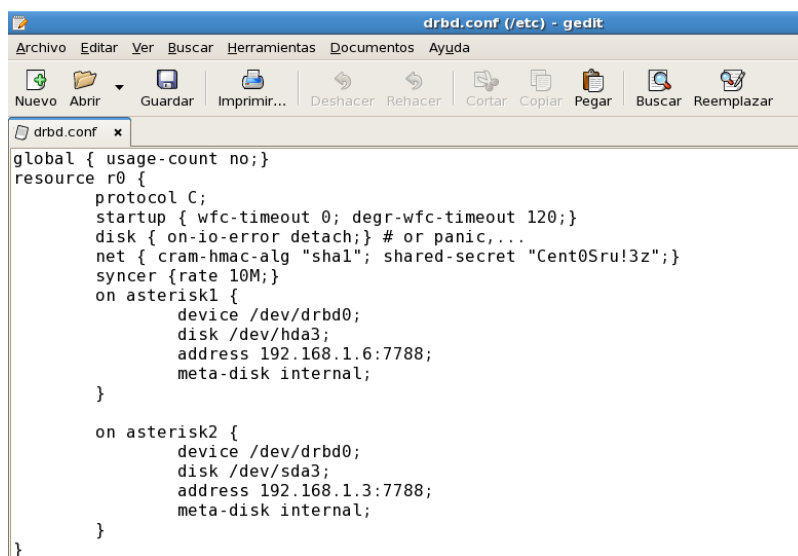
Fig. 4 Archivo /etc/drbd.conf
