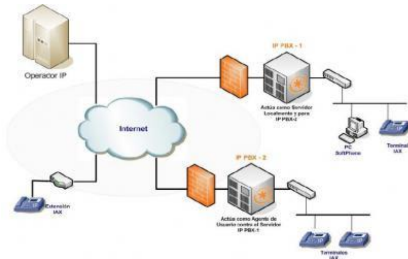
Figura 8 Protocolo IAX
