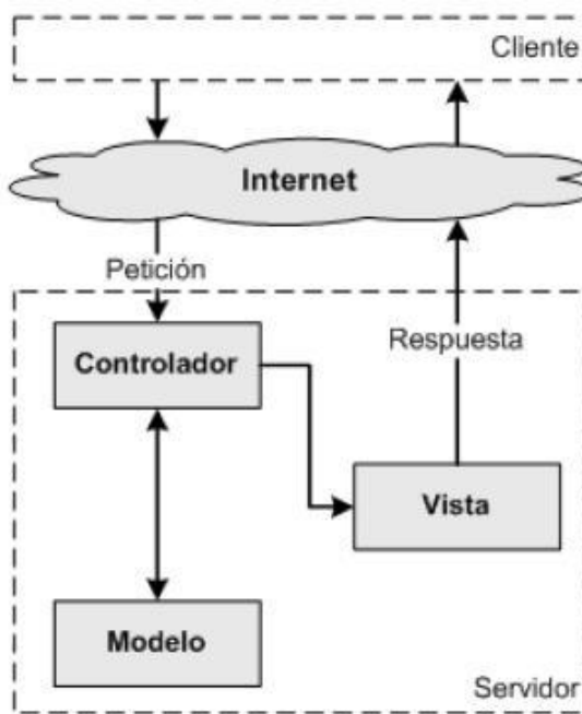
Figura 3.1: Diagrama de Arquitectura MVC.
