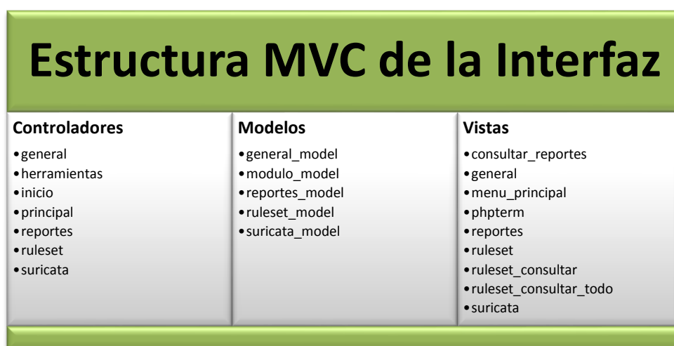
Figura 3.3 Estructura MVC de la Interfaz
