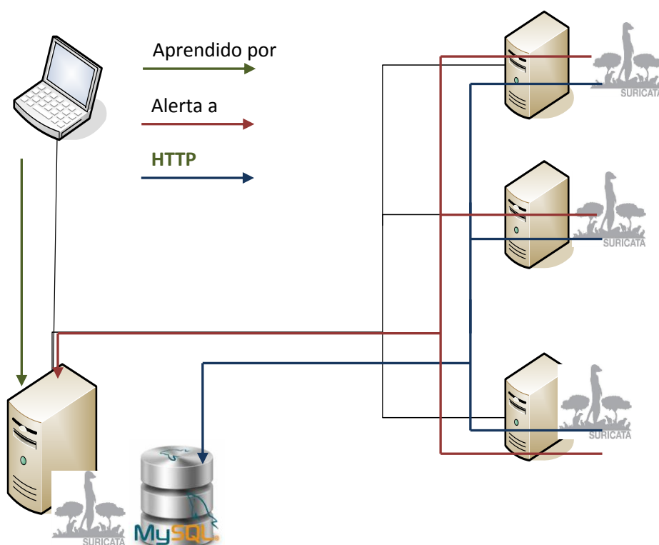
Figura 6.2: Diagrama Web Service para una interfaz centralizada
