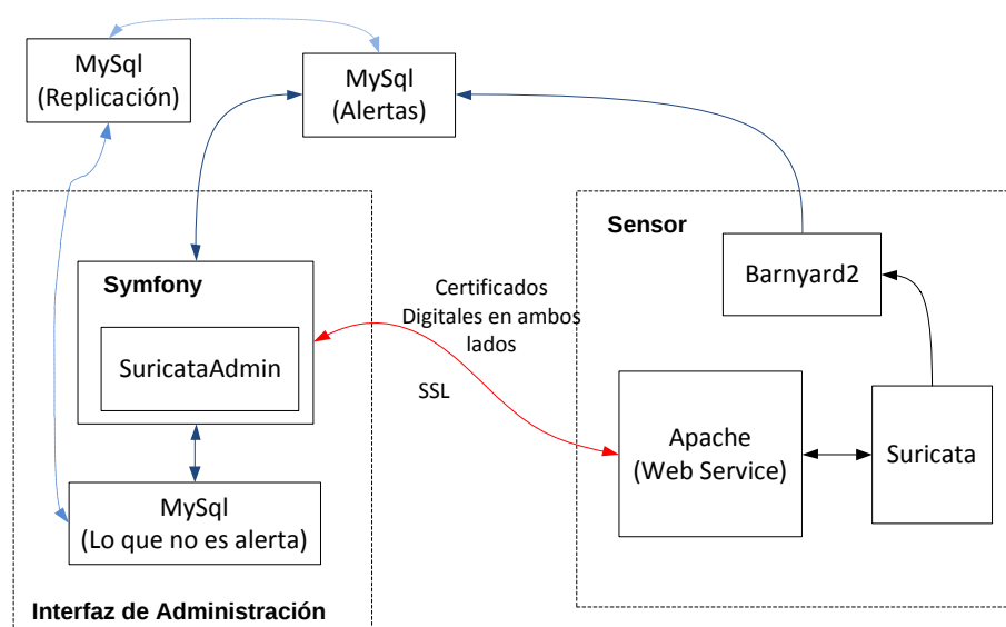
Figura 6.1: Diagrama de bloques para una interfaz centralizada
