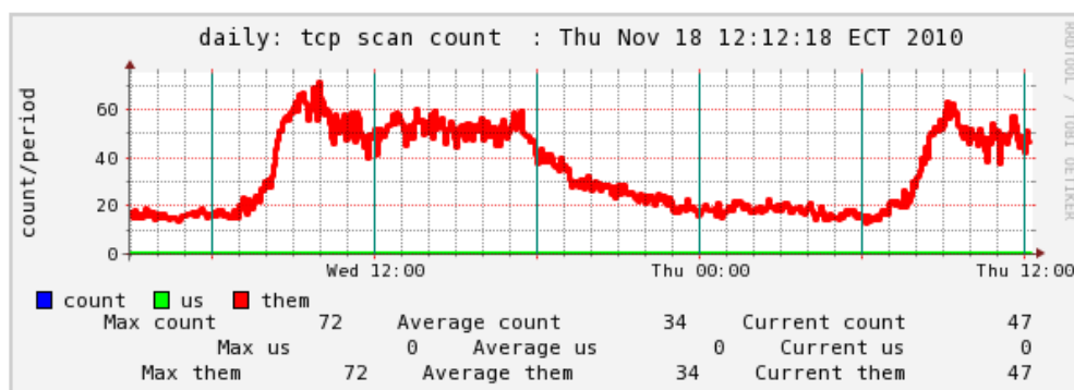
Figura 5.7 Grafo de detección de gusanos utilizando Ourmon.
