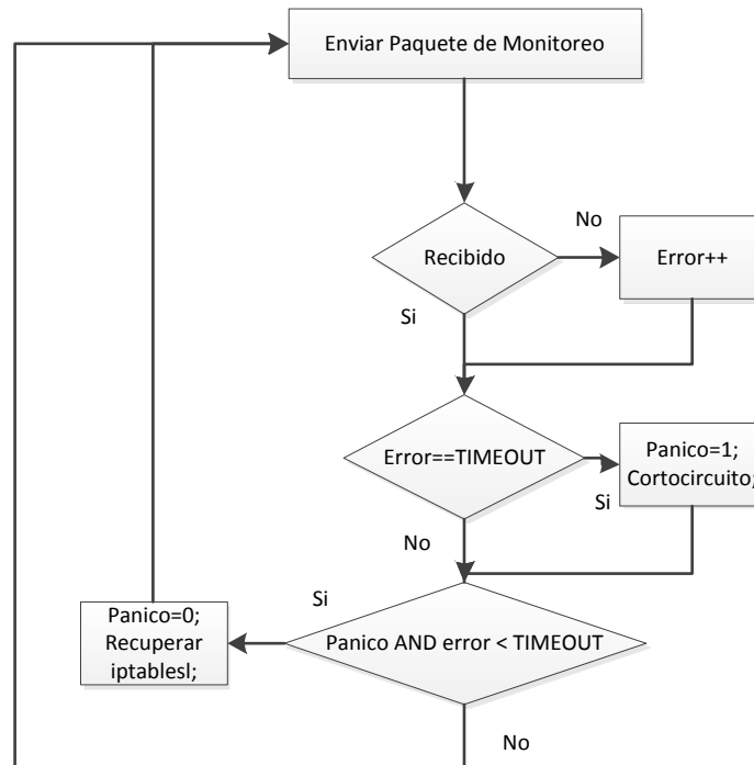
Figura 3.15 Diagrama de estados del módulo de recuperación de fallos
