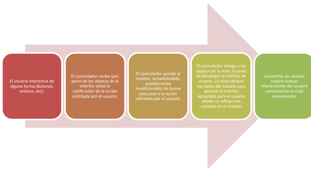
Figura 3.2: Proceso de la arquitectura Modelo Vista Controlador (MVC)
