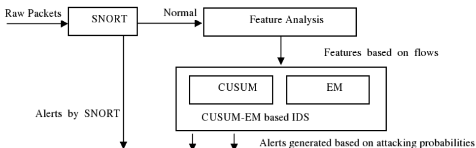
Figura 4.1 Arquitectura general del módulo de detección de anomalías.
