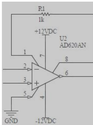
Figura 2.4.- Amplificador de instrumentación
