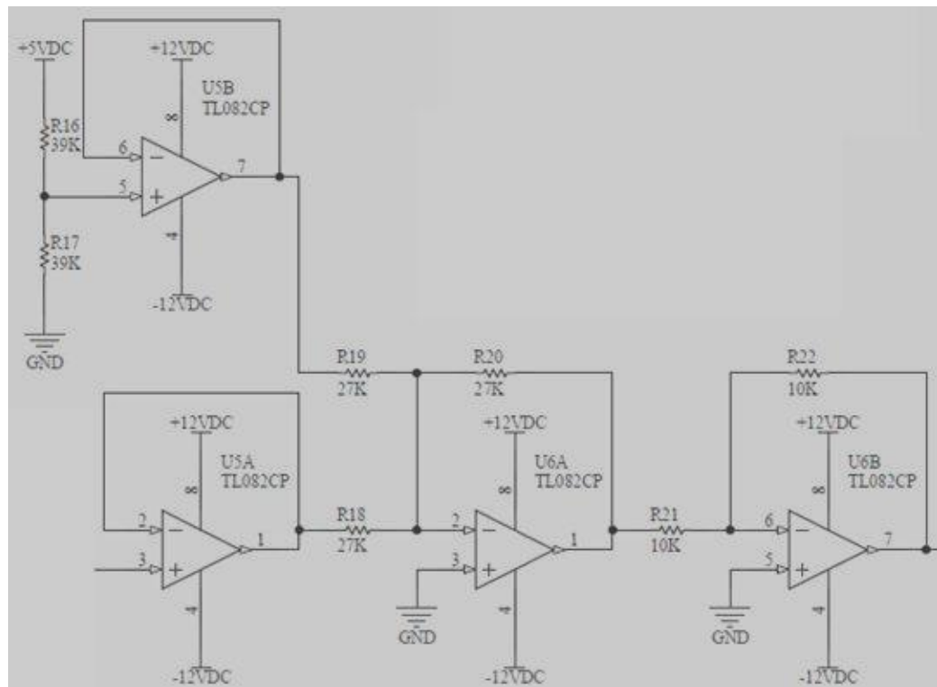
Figura 2.9.- Acondicionamiento de señales
