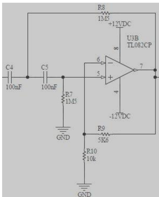
Figura 2.6.- Filtro pasa-altos
