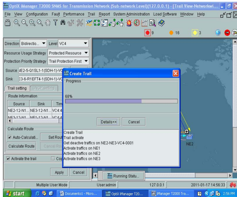
Figura 3.37 Configuración de Parámetros del Servicio
