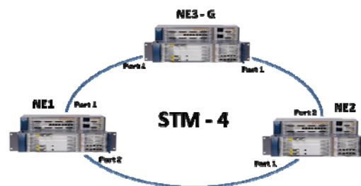
Figura 3.21 Conectividad entre los 3 Nodos
