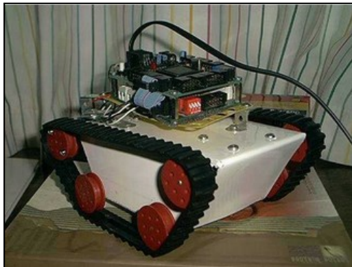
Fig. 1.4.3.1: Microbot SIKO
