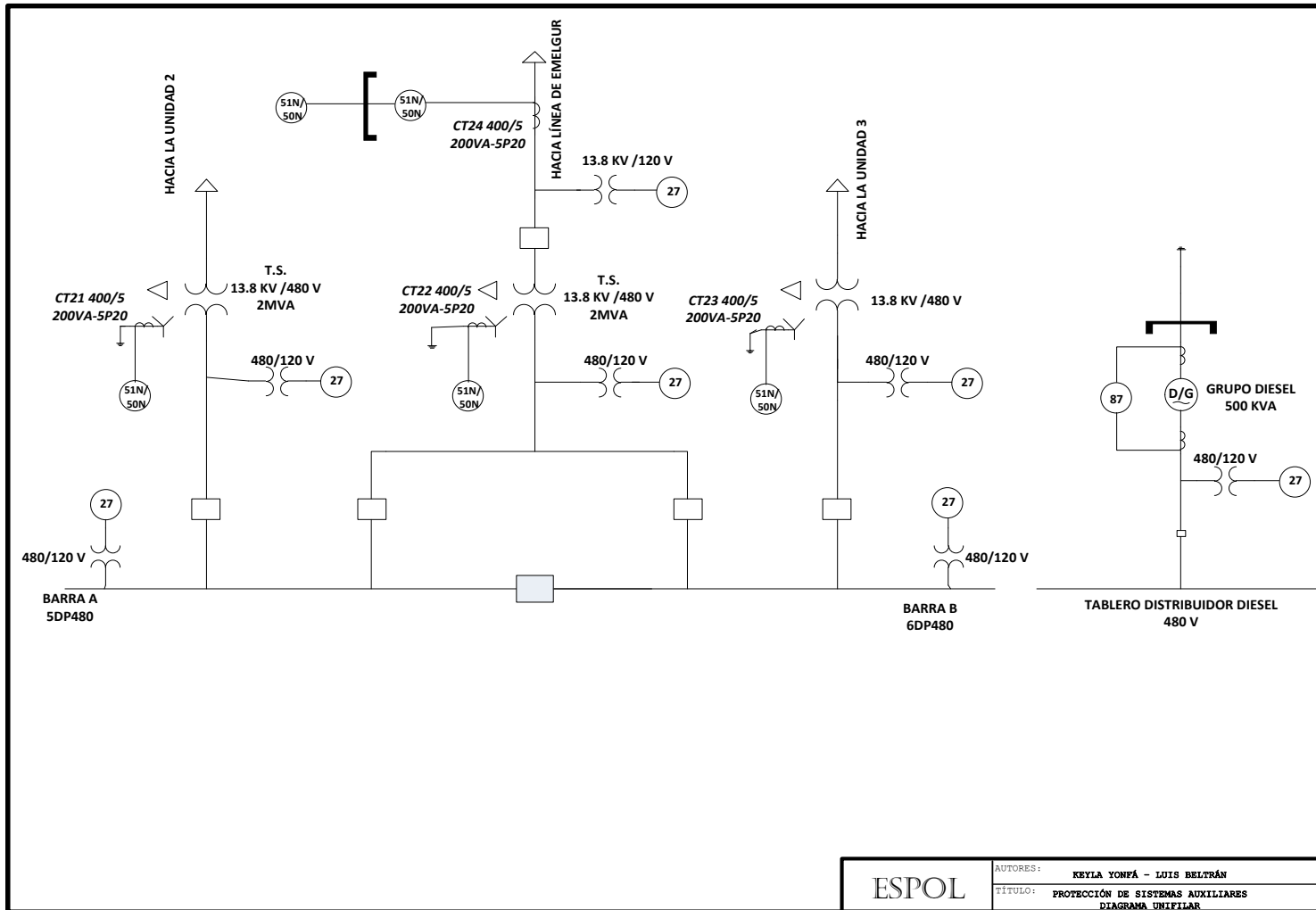
PAG. 4/5 ESQUEMA DE PROTECCIONES DE SERVICIOS AUXILIARES
