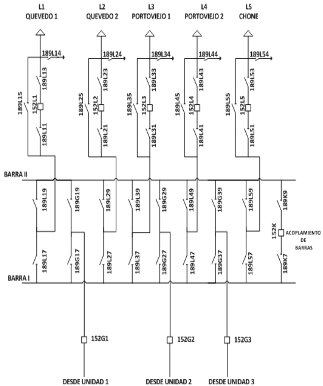
Figura 1.6 Diagrama Unifilar de la Subestación.
