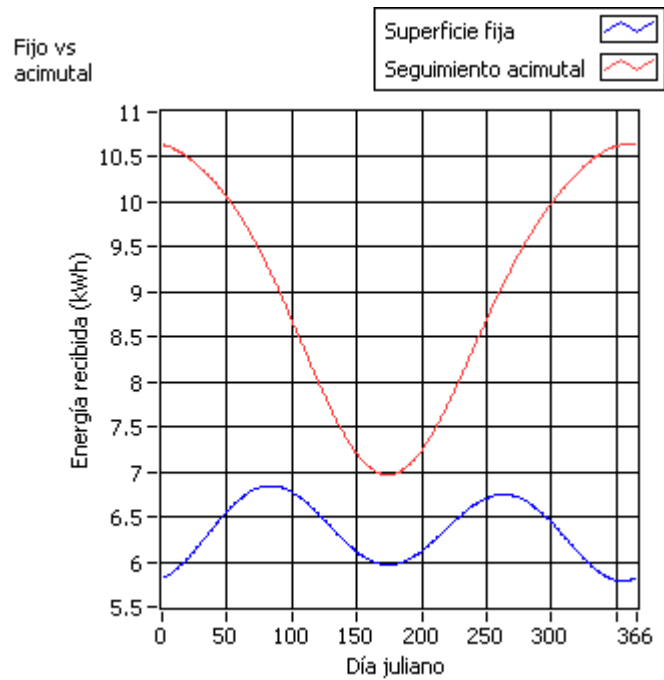
Figura 42.- Comparación fija vs. Acimutal en latitud 20° S
