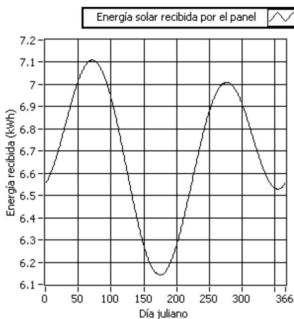
Figura 51.- Variación de la radiación en el sitio Maicito
