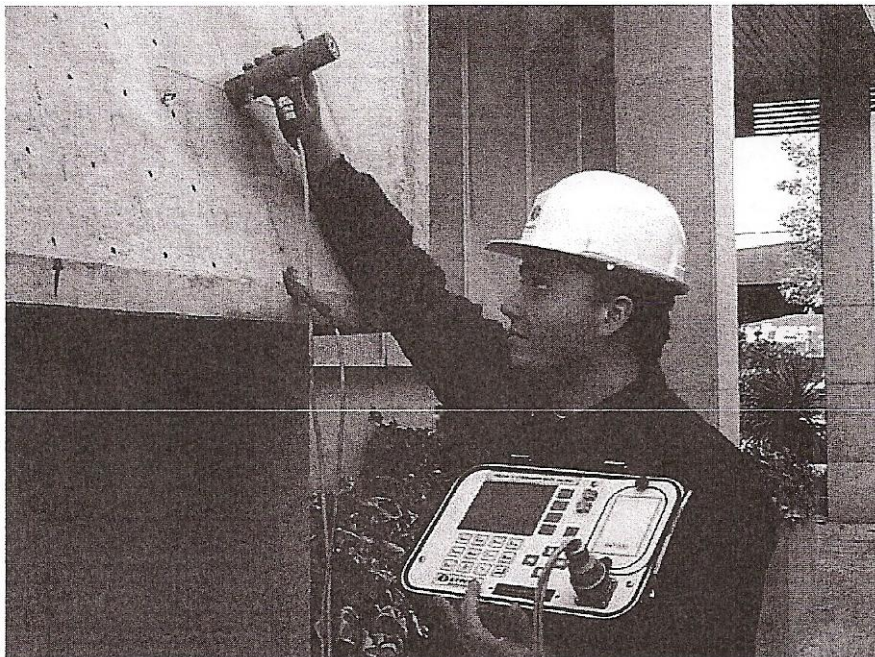
Figura 11 -. Dispositivo GECOR8 con sensor B
