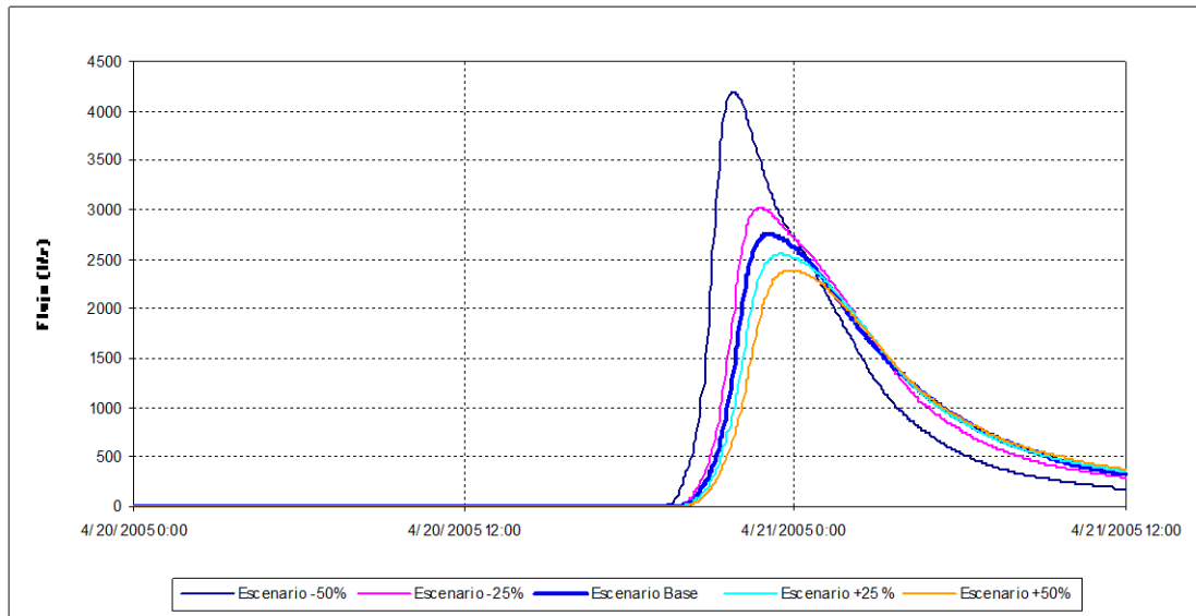
FIGURA 5.12 VARIACIONES DEL COEFICIENTE (N IMPERV)
