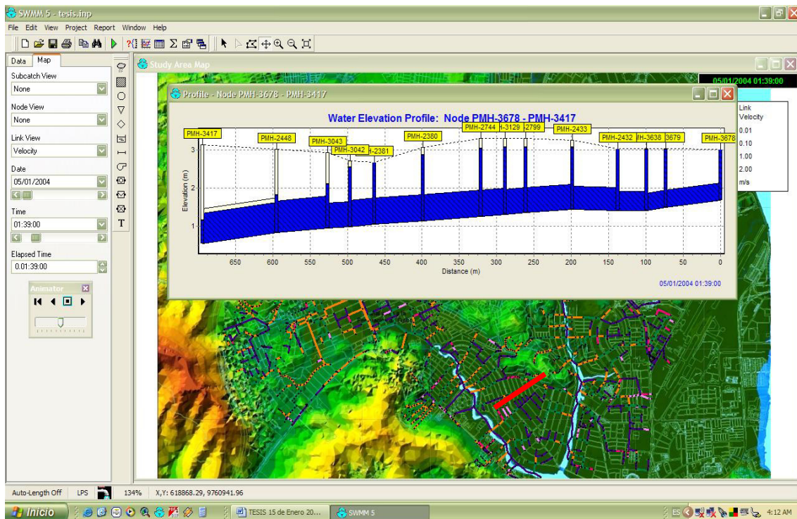
FIGURA 5.1 UBICACIÓN Y PERFIL LONGITUDINAL SUBCUENCA MIRAFLORES
