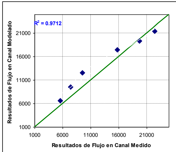
FIGURA 5.17 AJUSTE LINEAL DEL MODELO CALIBRADO.
