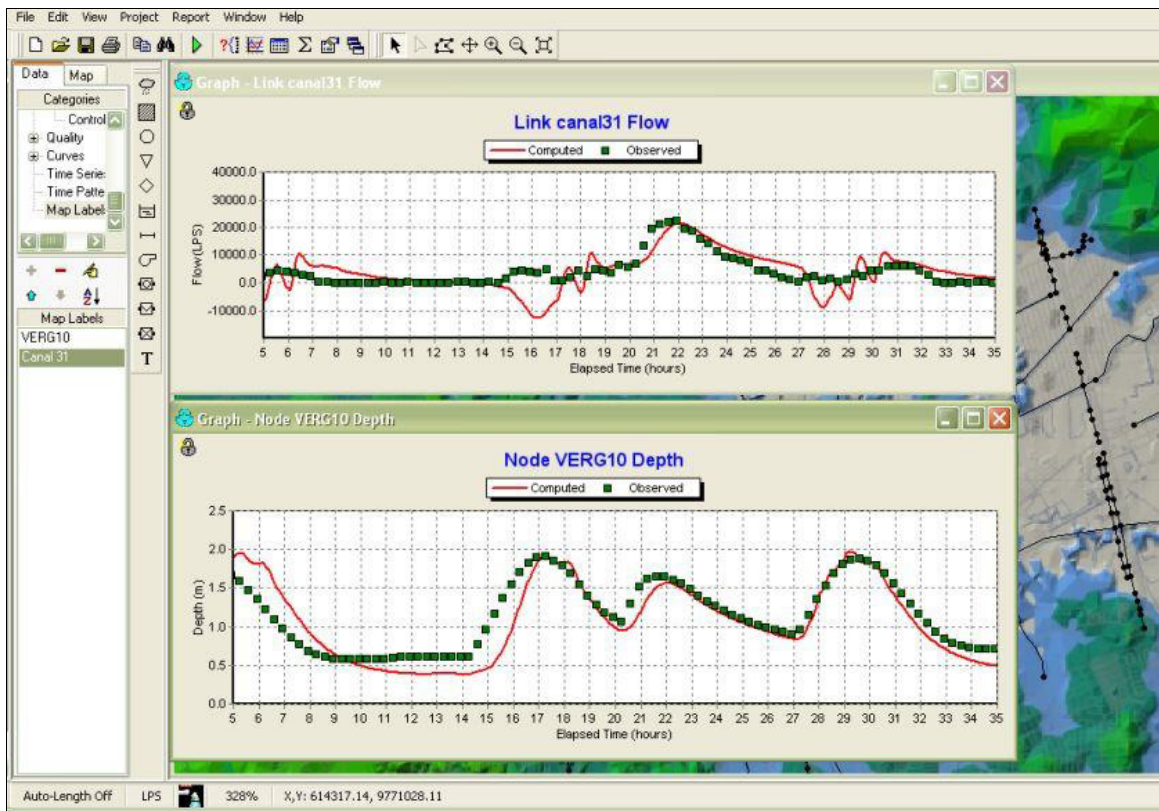
FIGURA 5.16 MODELO CALBRADO
