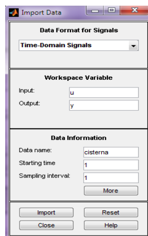
Figura 4-4.- Importar datos
