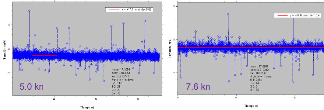
Figura No. 73 Resultados de Resistencia al Avance del Modelo con Flaps a 5° con Condición de Carga 1
