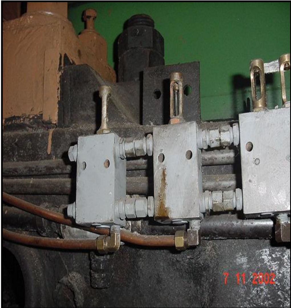
FIGURA 2.5 VALVULA DE MEDICION
