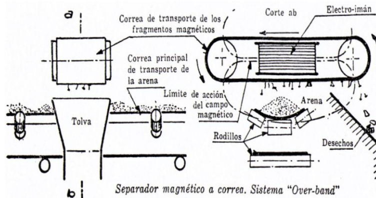
FIGURA 1.8 SEPARADOR MAGNÉTICO.
