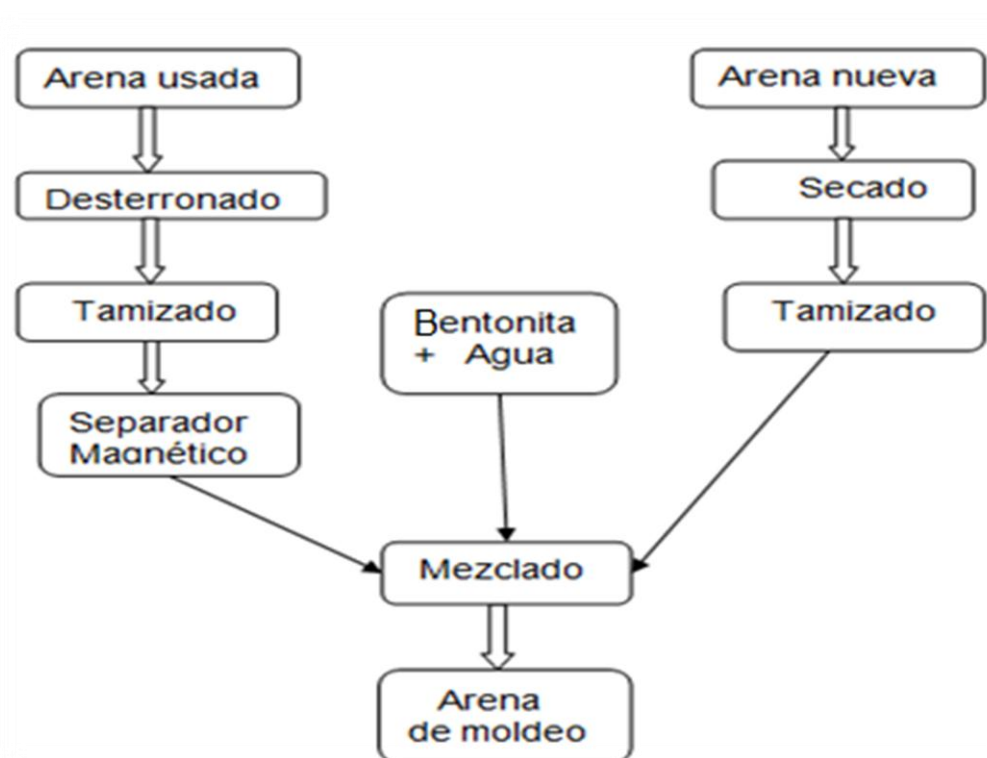
FIGURA 1.1 FLUJOGRAMA PREPARACIÓN DE ARENAS DE MOLDEO
