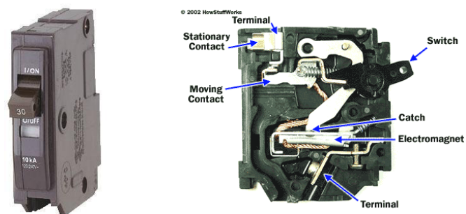
Figura 70. Vista de la palanca de un interruptor termo magnético (breaker)
