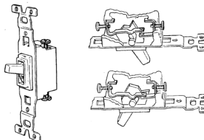
Figura 55. Interruptor silencioso.
