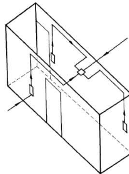
Figura 76. Alambrado de un pasillo con lámpara controlada desde dos posiciones.
