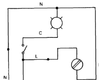
Figura 83 c). Diagrama esquemático.
