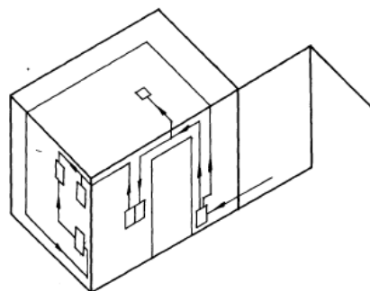
Figura 77. Alambrado de un baño.
