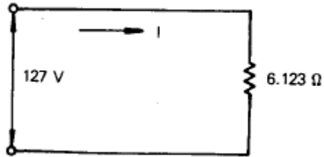
Figura 31. Circuito equivalente.
