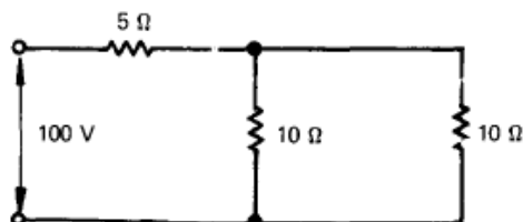
Figura 34. Resistencia equivalente del circuito.
