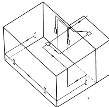
Figura 75. Alumbrado de una recamara con closet.
