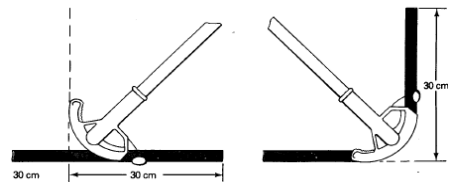
Doblado de tubo conduit a 90°
