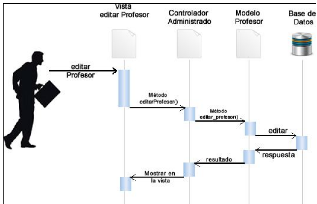
Figura XV: DIO 15 editar profesor.
