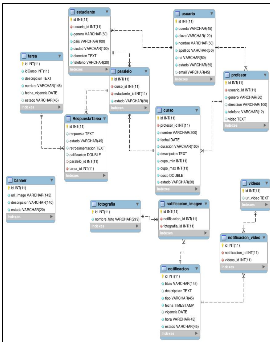
Figura XL: Modelo de base de datos.
