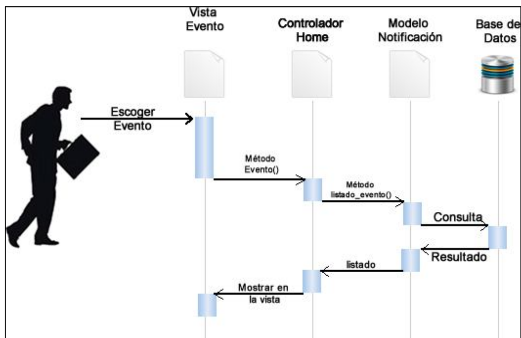
Figura V: DIO 5 Escoger evento
