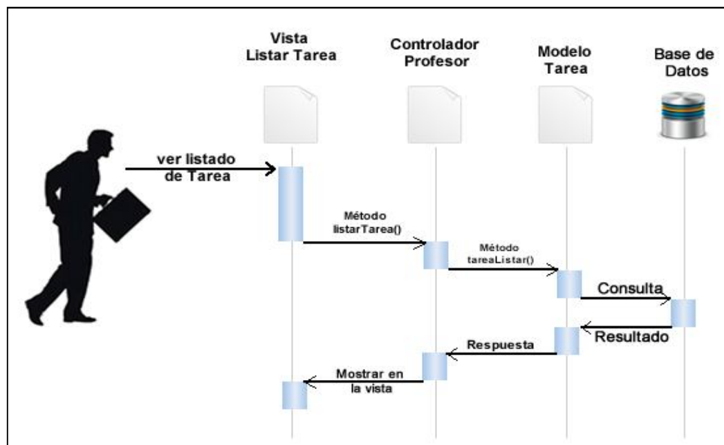
Figura XXXII: DIO 33 Ver listado de tareas respondidas.
