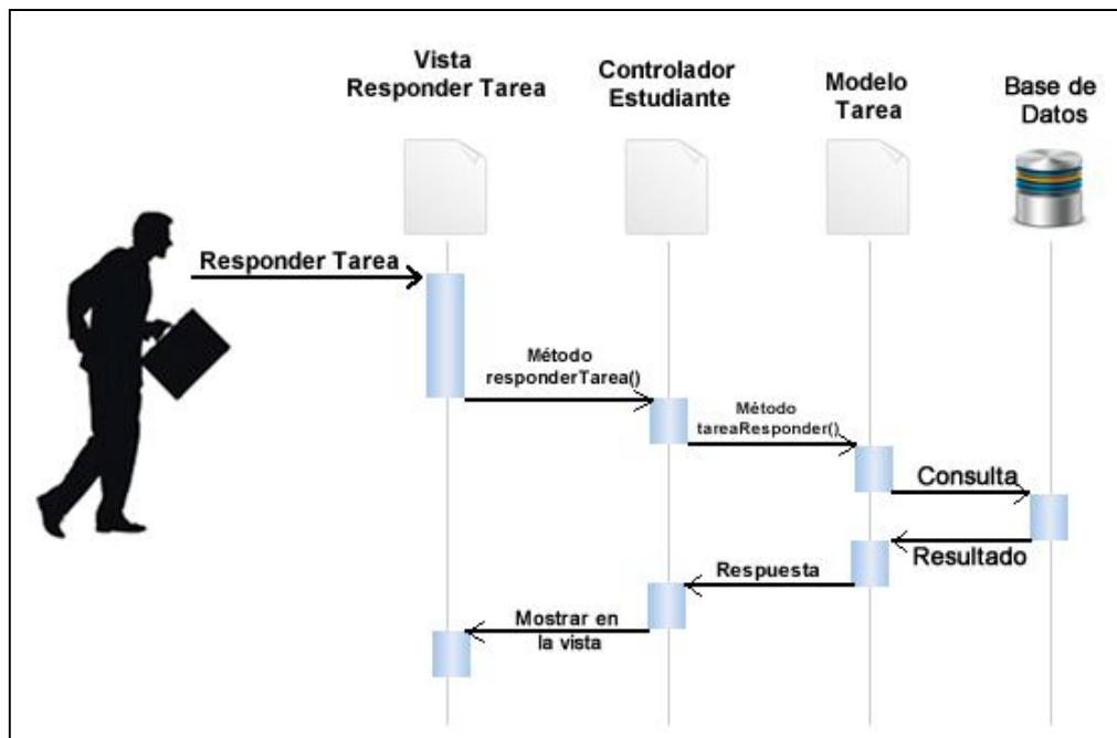
Figura XXVII: DIO 27 Editar respuesta tarea.
