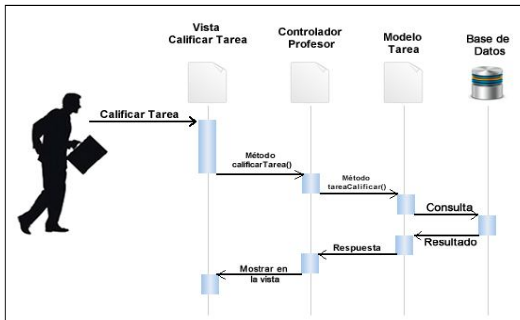
Figura XXXV: DIO 36 Recalificar Tarea.
