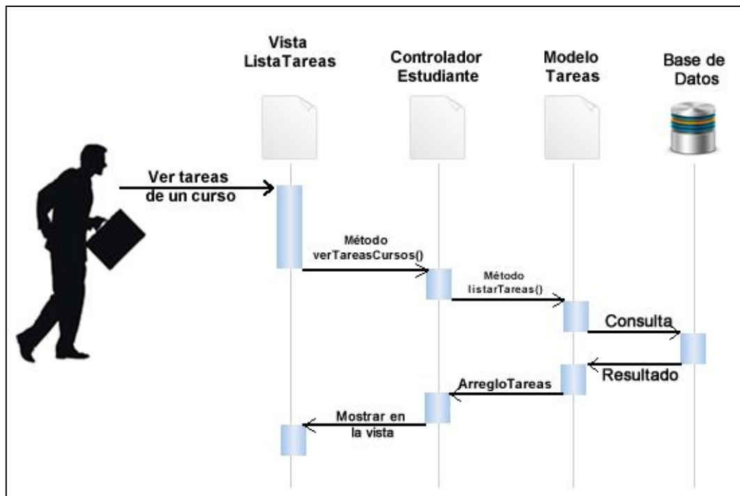
Figura XXIII: DIO Ver listado de Tareas
