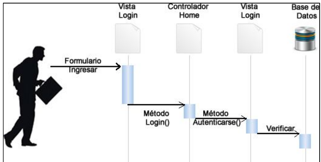
Figura I: DIO 1 Ingreso al sistema
