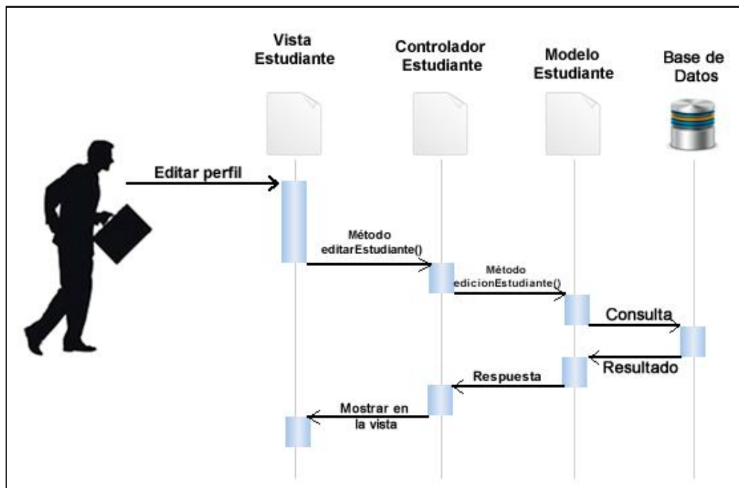
Figura XXVIII: DIO 29 Editar perfil estudiante.
