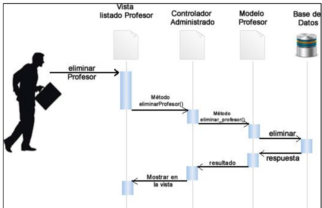
Figura XVI: DIO 16 eliminar profesor.
