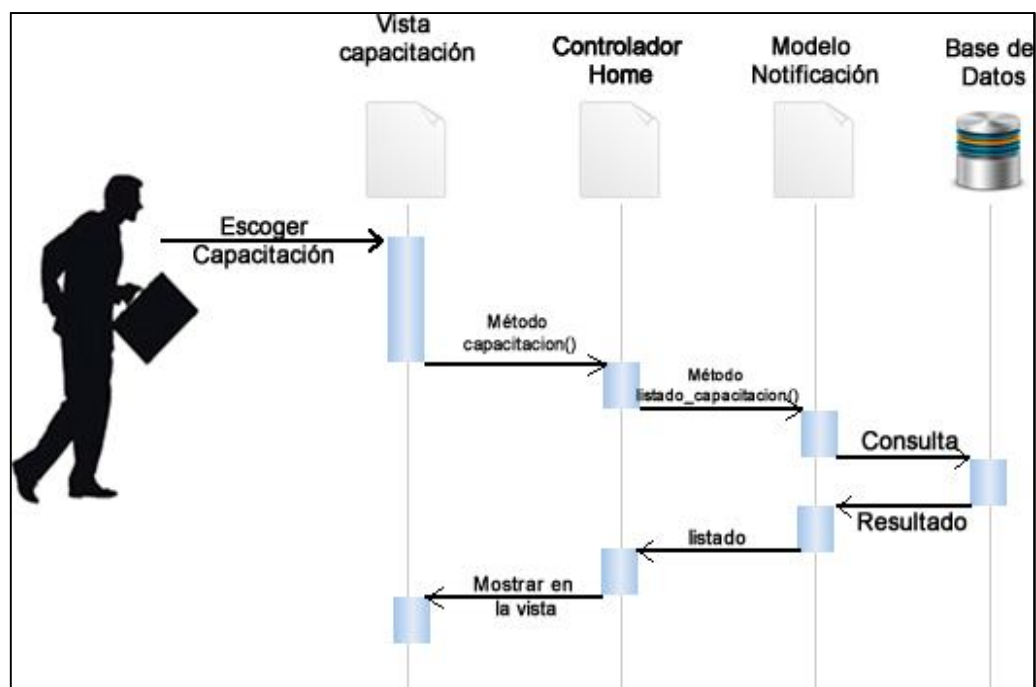
Figura VI: DIO 6 escoger capacitación.
