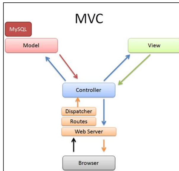
Figura XXXVII: Esquema referente al MVC. [2]
