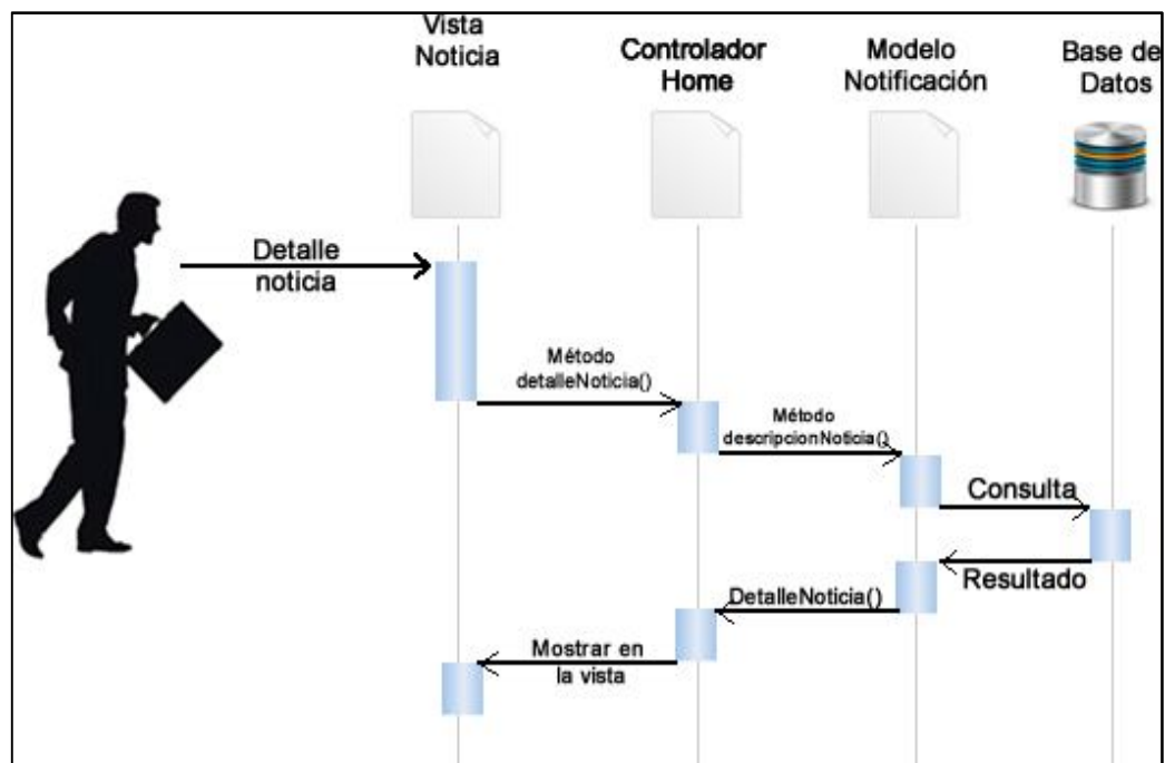
Figura VII: DIO 7 ver detalle noticia.
