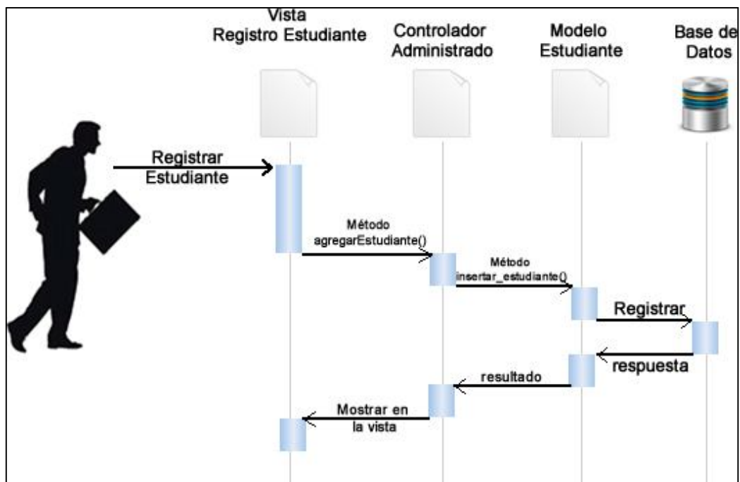
Figura XIII: DIO 13 registro estudiante.
