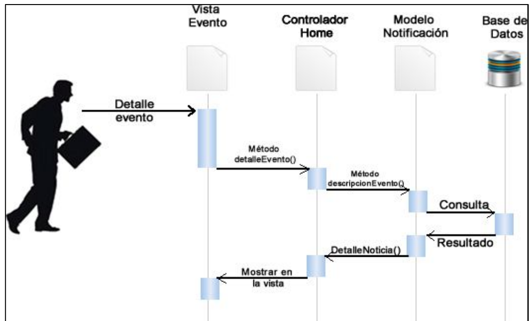
Figura VIII: DIO 8 ver detalle evento.
