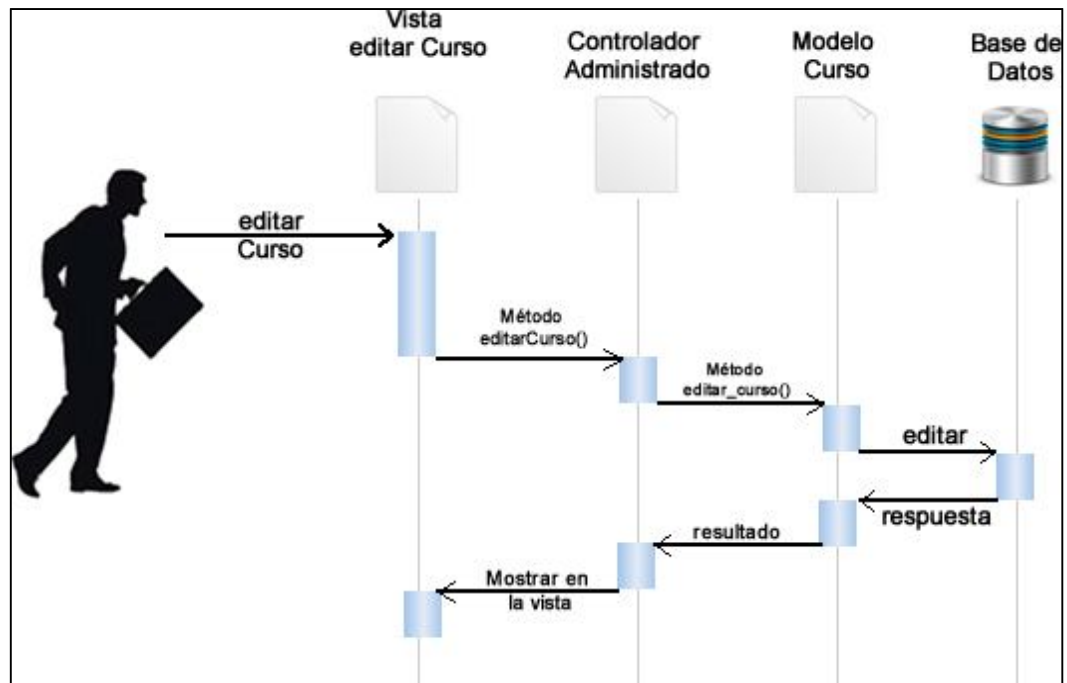
Figura XIX: DIO 19 Editar cursos.
