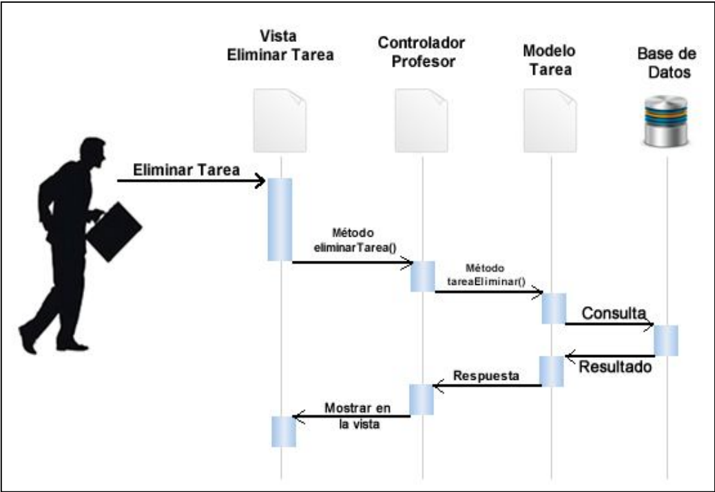
Figura XXV: DIO 25 Eliminar Tarea.
