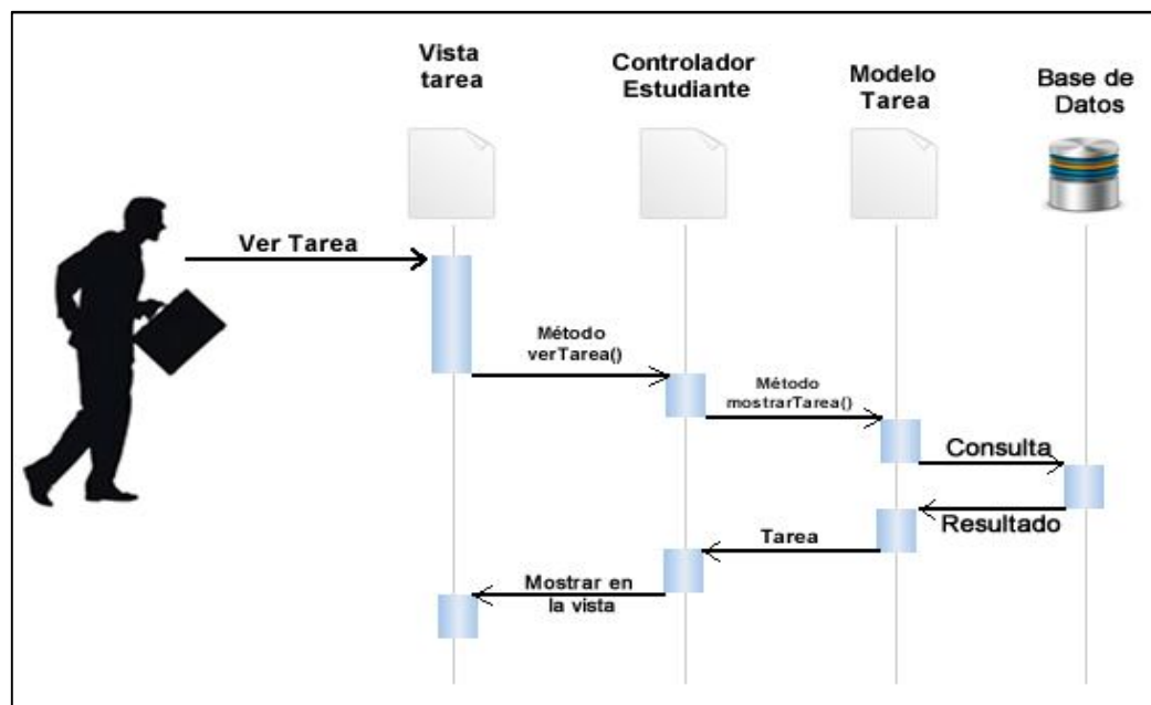
Figura XXIV: DIO 24 Ver Tarea.
