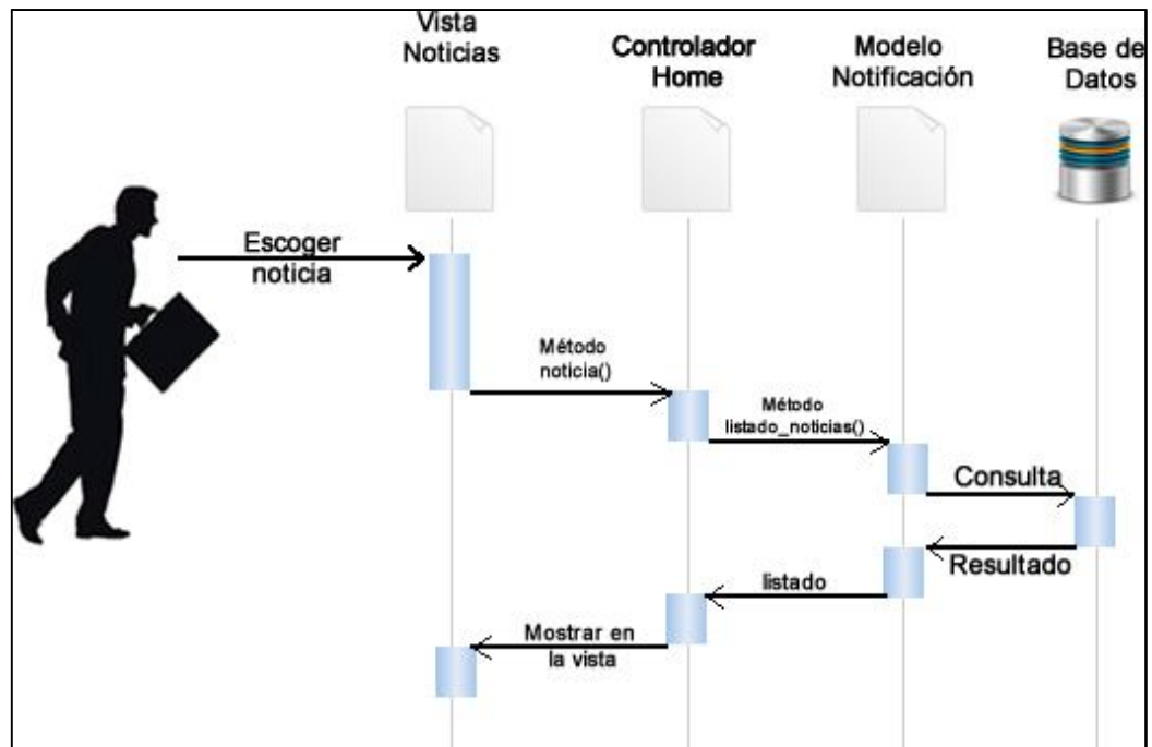
Figura IV: DIO 4 Escoger noticia
