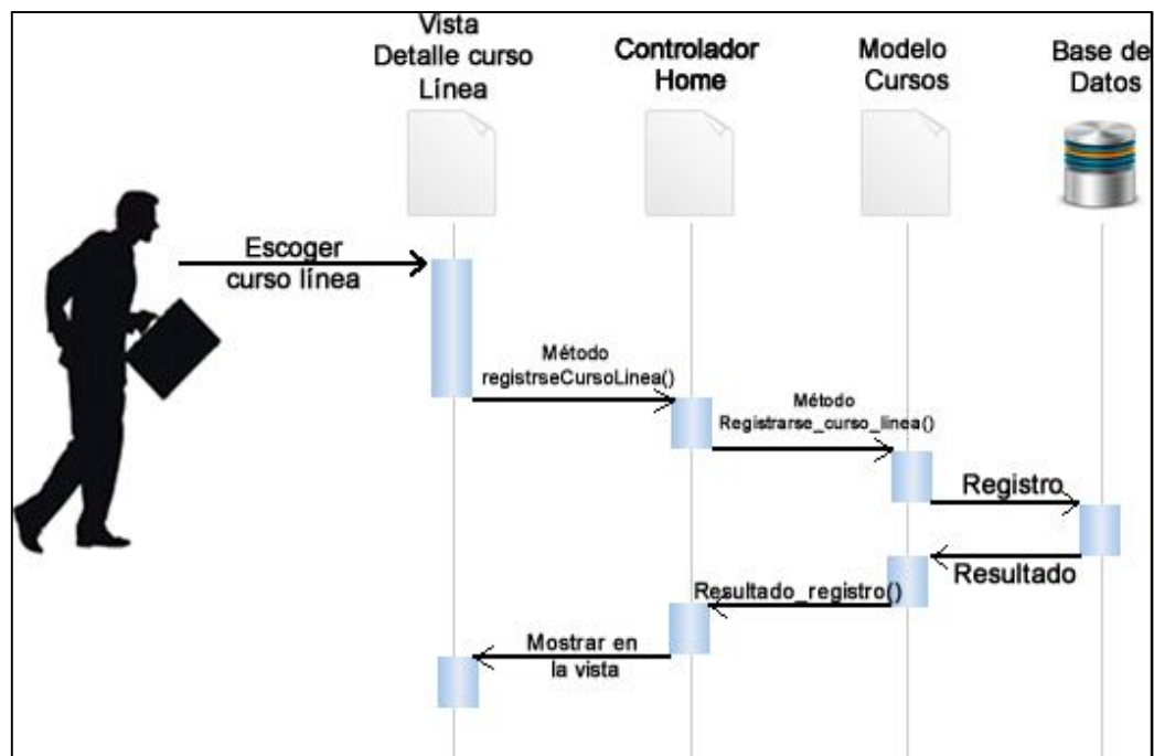
Figura III: DIO 3 escoger curso en línea
