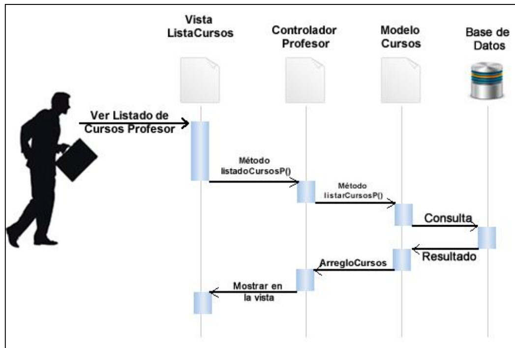
Figura XXXI: DIO 32 Ver listado de Cursos.
