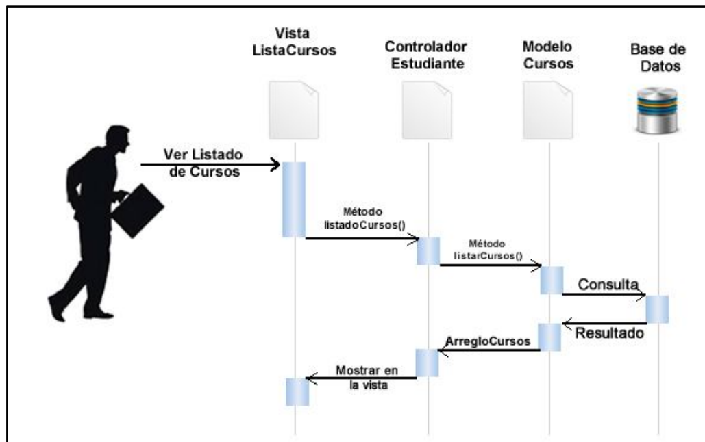
Figura XXII: DIO 22 Ver listado de Cursos
