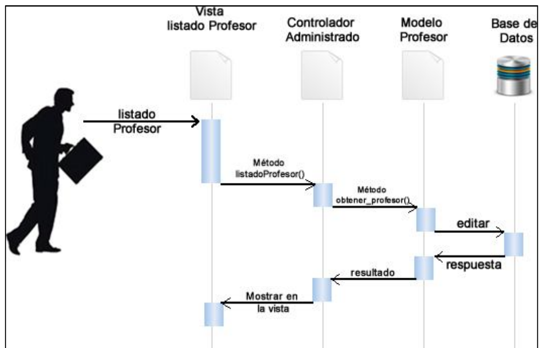
Figura XIV: DIO 14 Listado profesor.
