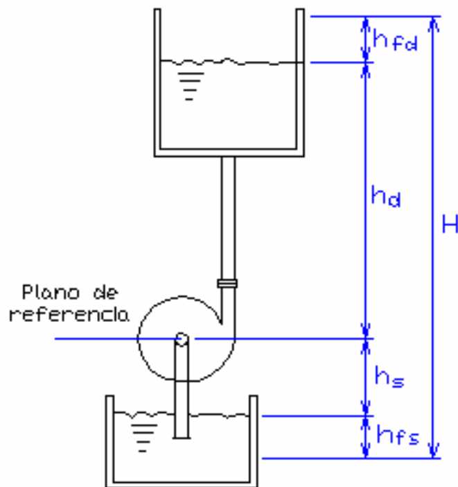
FIGURA 1. VARIABLES PARA EL CALCULO DE LA CARGA DE BOMBA
