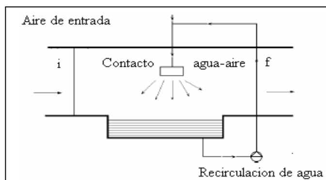
FIGURA 1.11 ENFRIAMIENTO EVAPORATIVO
