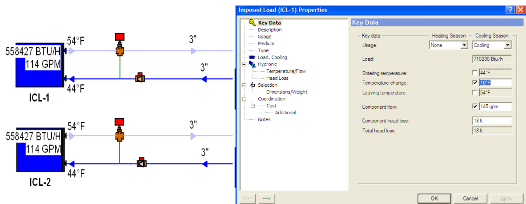
FIGURA 3.12, DISEÑO EN SERPENTINES DE ENFRIAMIENTO E INGRESO DE DATOS
