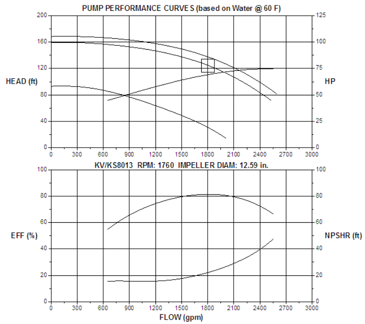
FIGURA 3.7, CURVA DE SELECCIÓN DE BOMBA PRIMARIA
