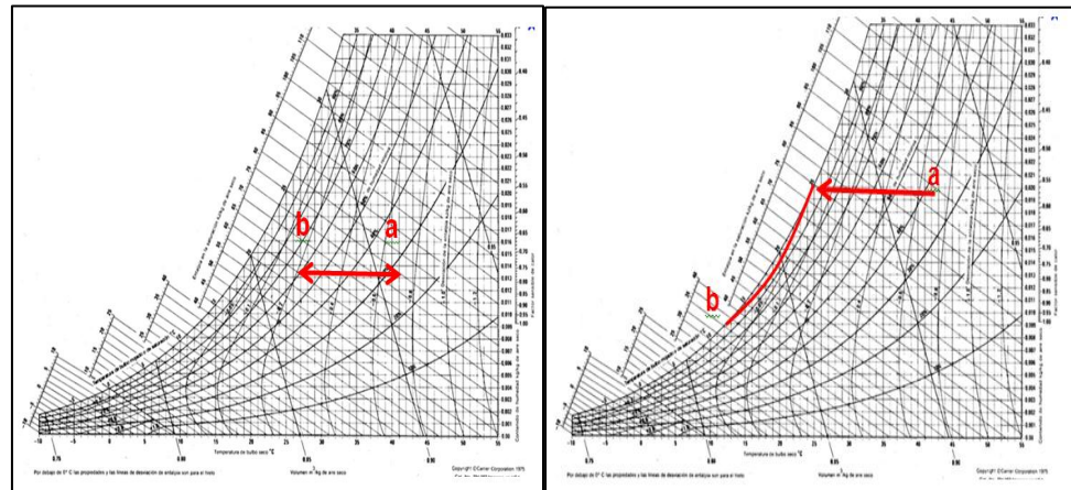
FIGURA 1.14 PROCESO DE ENFRIAMIENTO POR COMPRESIÓN MECÁNICA
