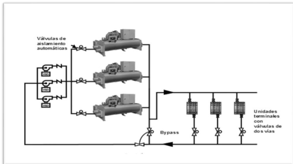
FIGURA 3.4 SISTEMA PRIMARIO VARIABLE
