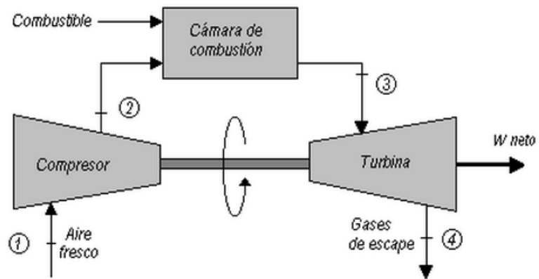
FIGURA 1.3 FUNCIONAMIENTO Y PARTES DE UNA TURBINA A GAS SIMPLE
