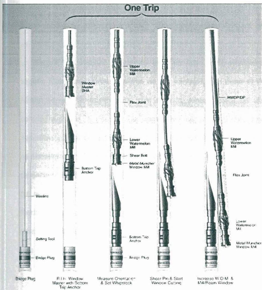
FIGURA 3.2 BHA PARA ABRIR VENTANA
