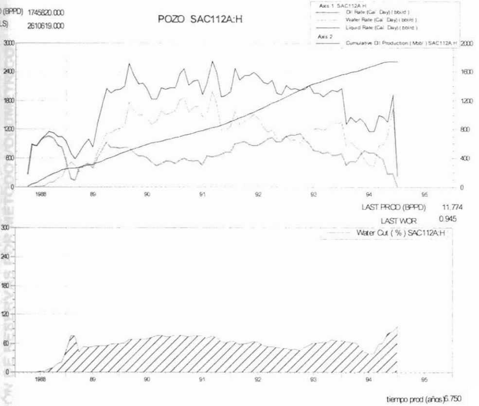
FIGURA 1.4 DECLINACION DEL POZO SACHA 112
