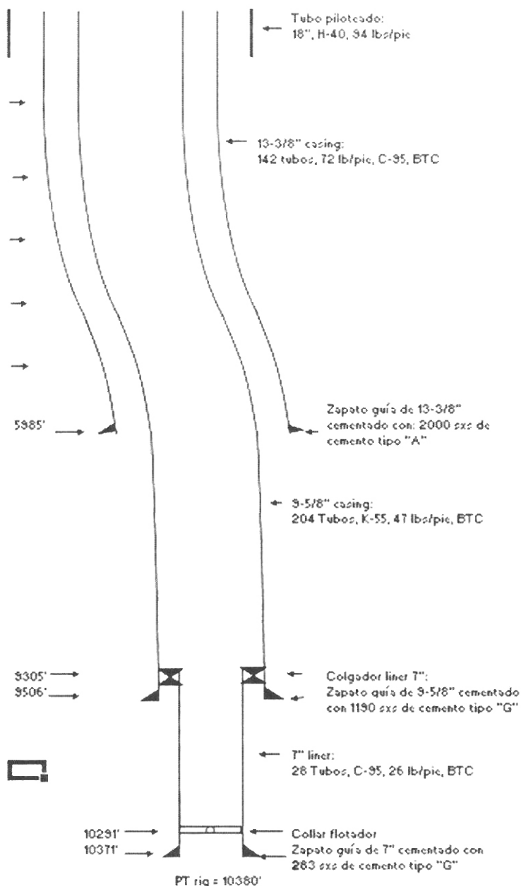
FIGURA 3.9 DIAGRAMA DE PERFORACION POZO SACHA 225
