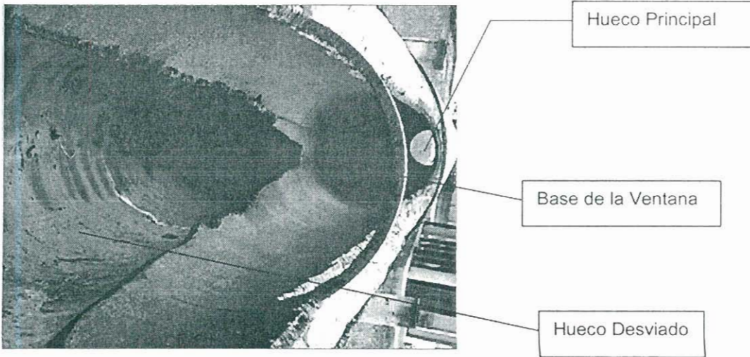
FIGURA 3.1 PERFIL DE UNA VENTANA (CORTE DE CASING)
