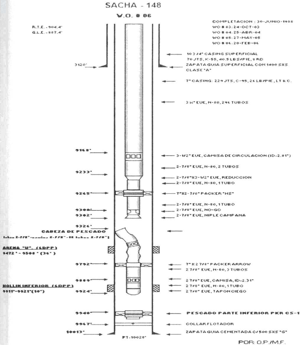
FIGURA 2.1 ESTADO MECANICO DEL POZO SACHA 148
