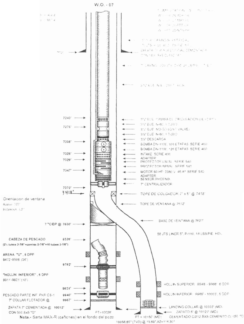
FIGURA 3.6 COMPLETACION FINAL DEL POZO SACHA 148
