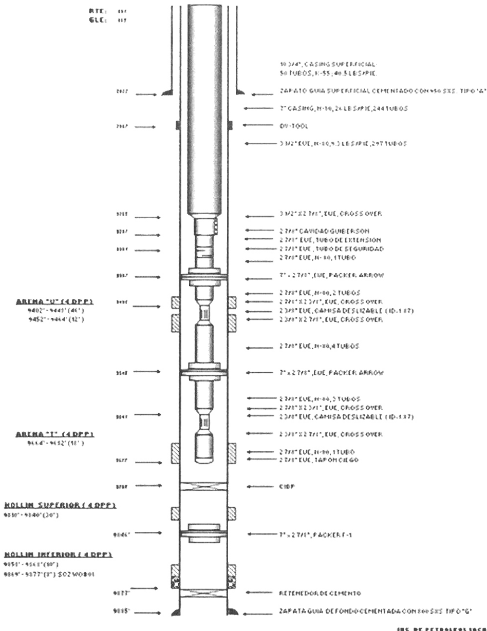
FIGURA 3.7 COMPLETACION FINAL DEL POZO SACHA 112
