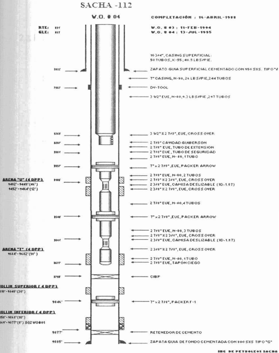
FIGURA 2.3 ESTADO MECANICO DEL POZO SACHA 112
