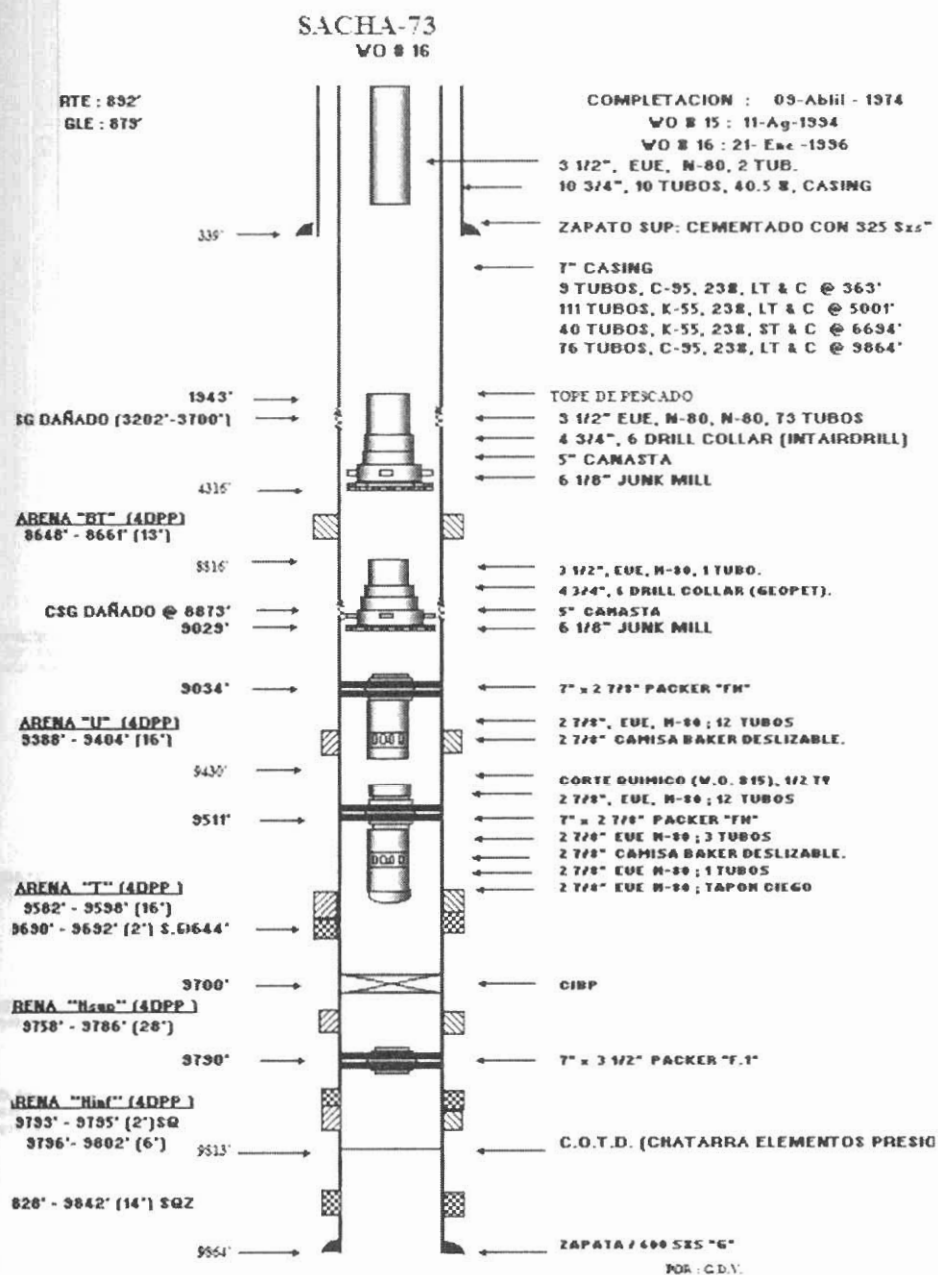
FIGURA 2.2 ESTADO MECANICO DEL POZO SACHA 73
