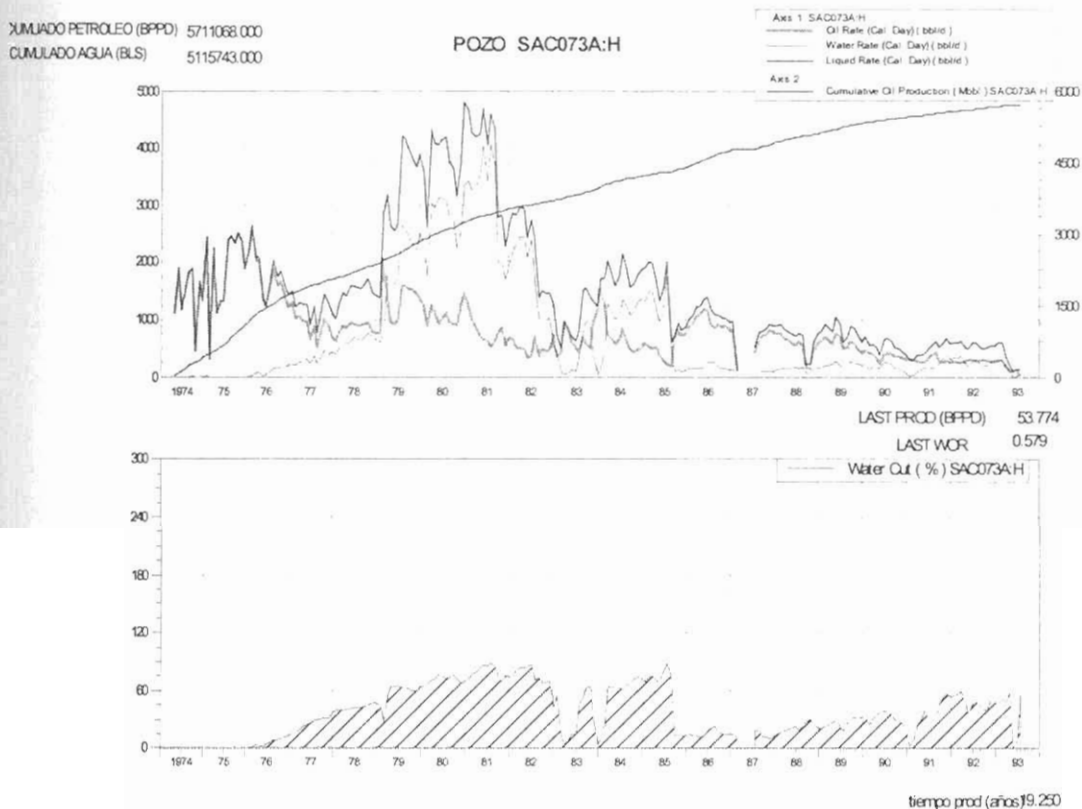
FIGURA 1.3 DECLINACION DEL POZO SACHA 73
