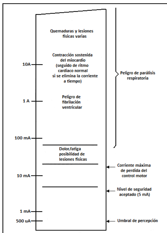
Figura 1. Efectos fisiológicos de la corriente eléctrica
