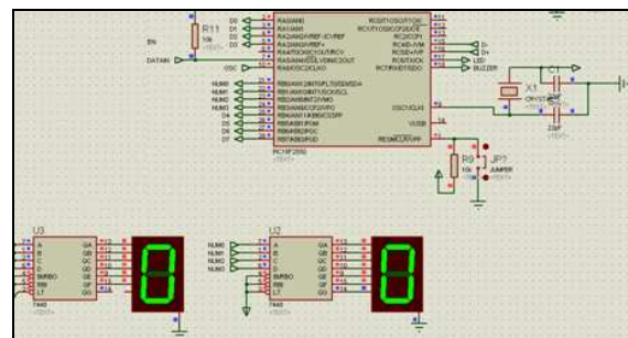
Figura 7. Simulación de los displays sin paso de corriente
