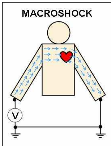
Figura 2. Ejemplo de macroshock
