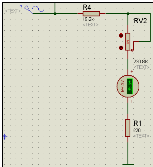
Figura 4. Simulación de la Etapa de Adquisición
