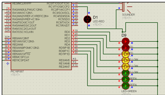
Figura 8. Simulación de los ocho niveles de leds activos
