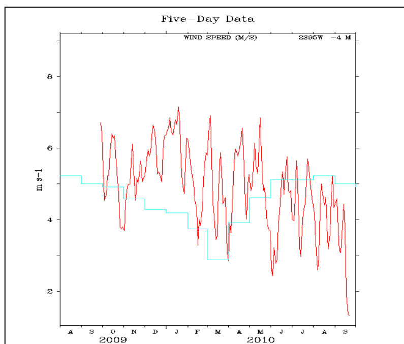
Figura 9. Velocidad de viento ( 2^{\circ} s 95^{\circ} w, h=4\text{m} )
