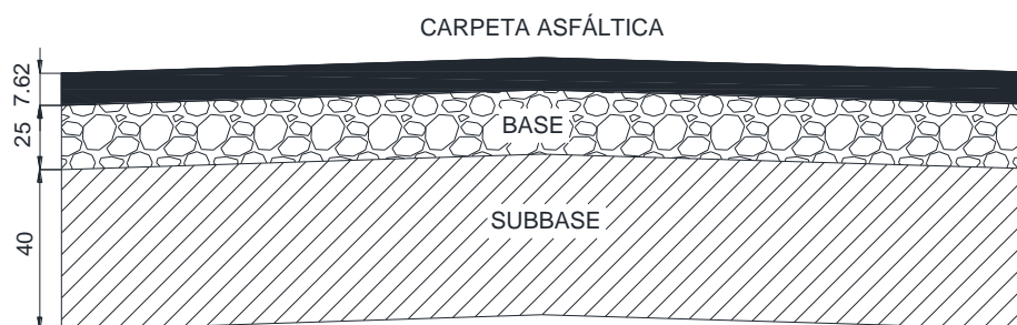
Figura 4.1 Sección Típica del Pavimento para la vía "Playa de Vinces – Bagatela".
