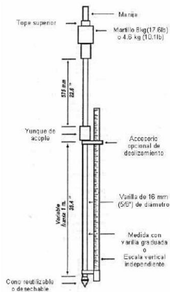
Figura 3.1 Configuración del Pentrómetro Dinámico de Cono
