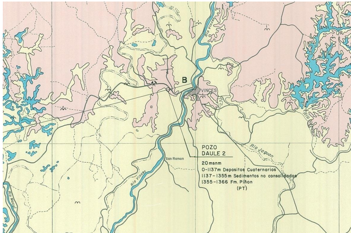
Figura 2.1 Mapa Geológico de la zona
