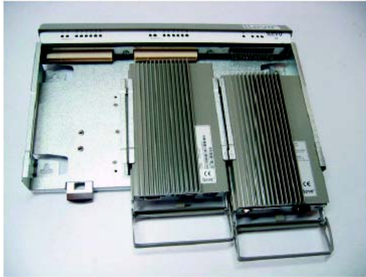
Figura 3-14 Módulos ILV22B2 con ILV22M2 y suministro de poder ILV22P1 [34]
