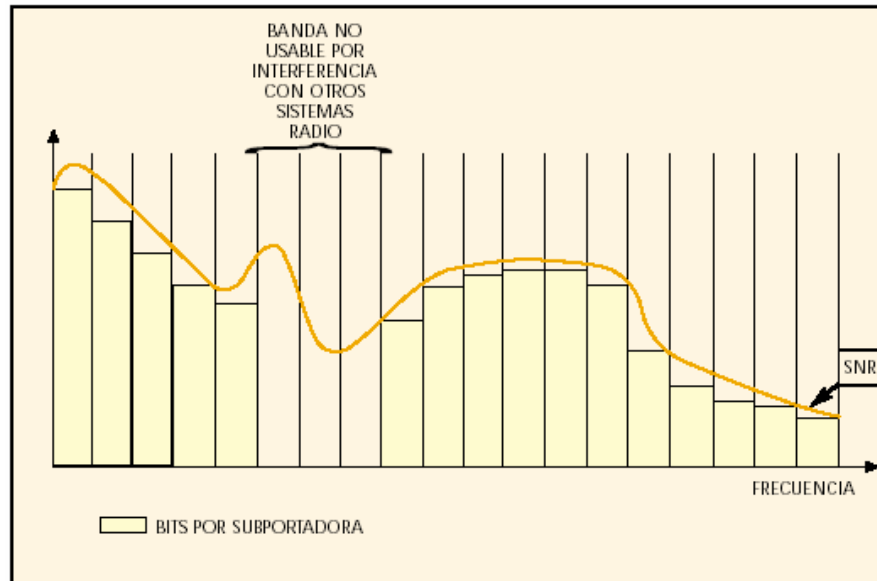
Figura 3-3 Subportadoras usadas para la transmisión de datos [29]
