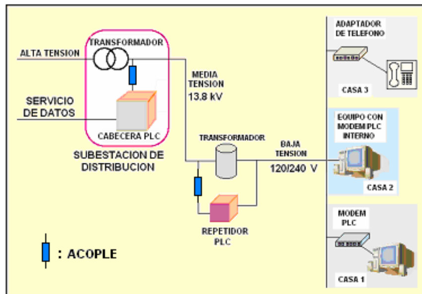
Figura 3-26 Esquema de la conexión resultante [38]
