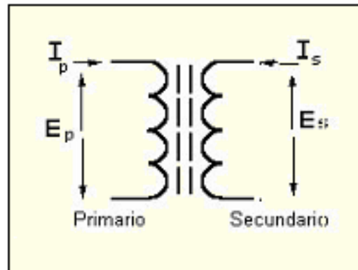
Figura 2-8 Diagrama esquemático del transformador [18]
