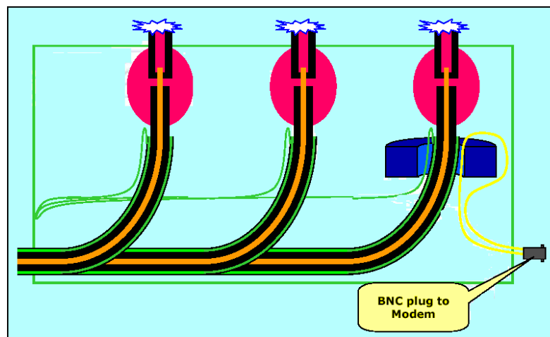
Figura 3-19 Modo de inserción fase-tierra del acople inductivo
