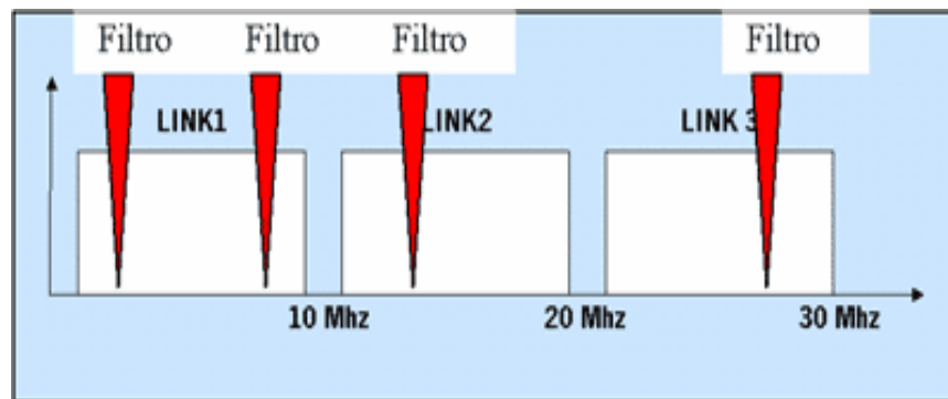
Figura 3-5 Sistema de modulación OFDM con filtros
