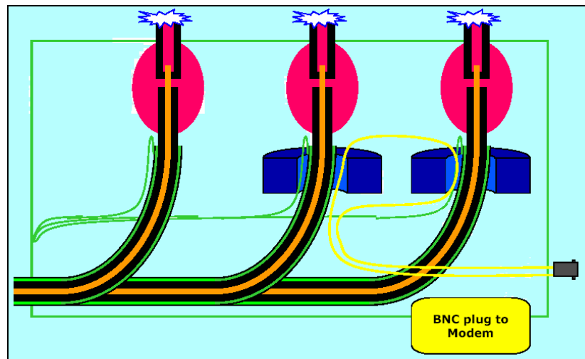
Figura 3-20 Modo de inserción fase-fase del acople inductivo
