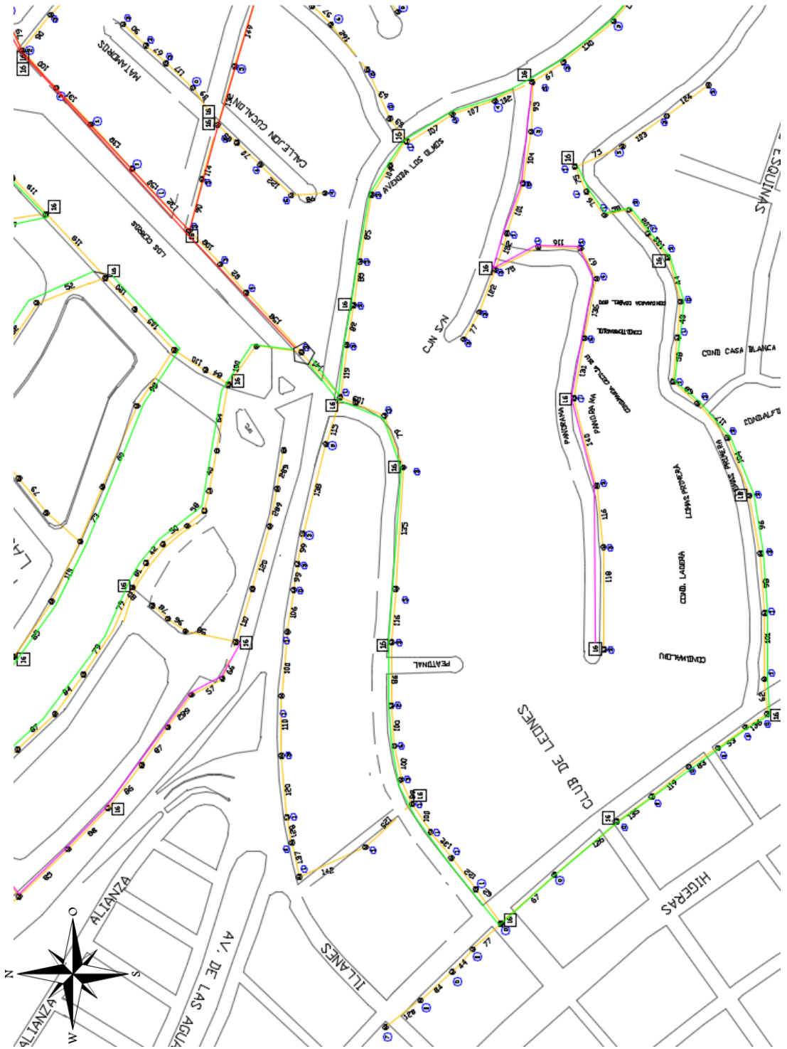
Figura 4.8 Diseño de la Red G-PON - Zona 4 Parte 2
