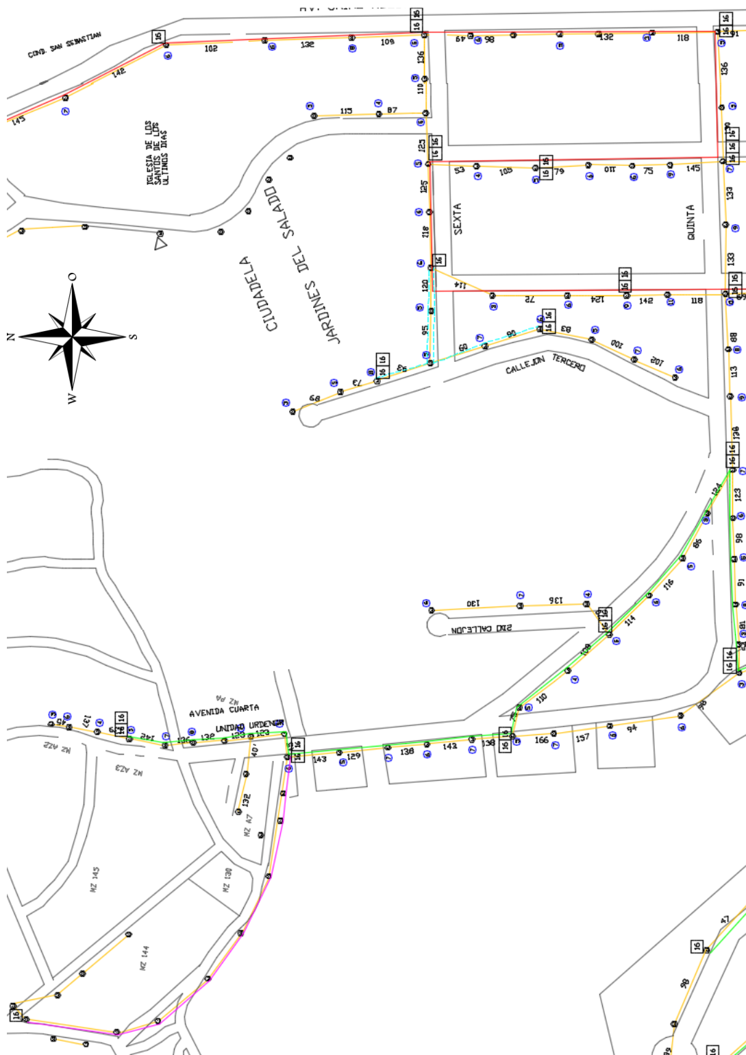
Figura 4.5 Diseño de la Red G-PON - Zona 2
