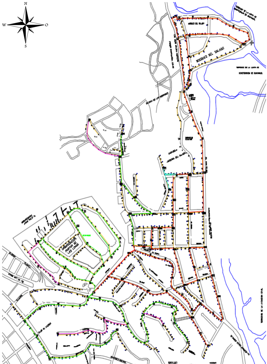
Figura 4.9 Diseño de la Red G-PON - Cobertura Total
